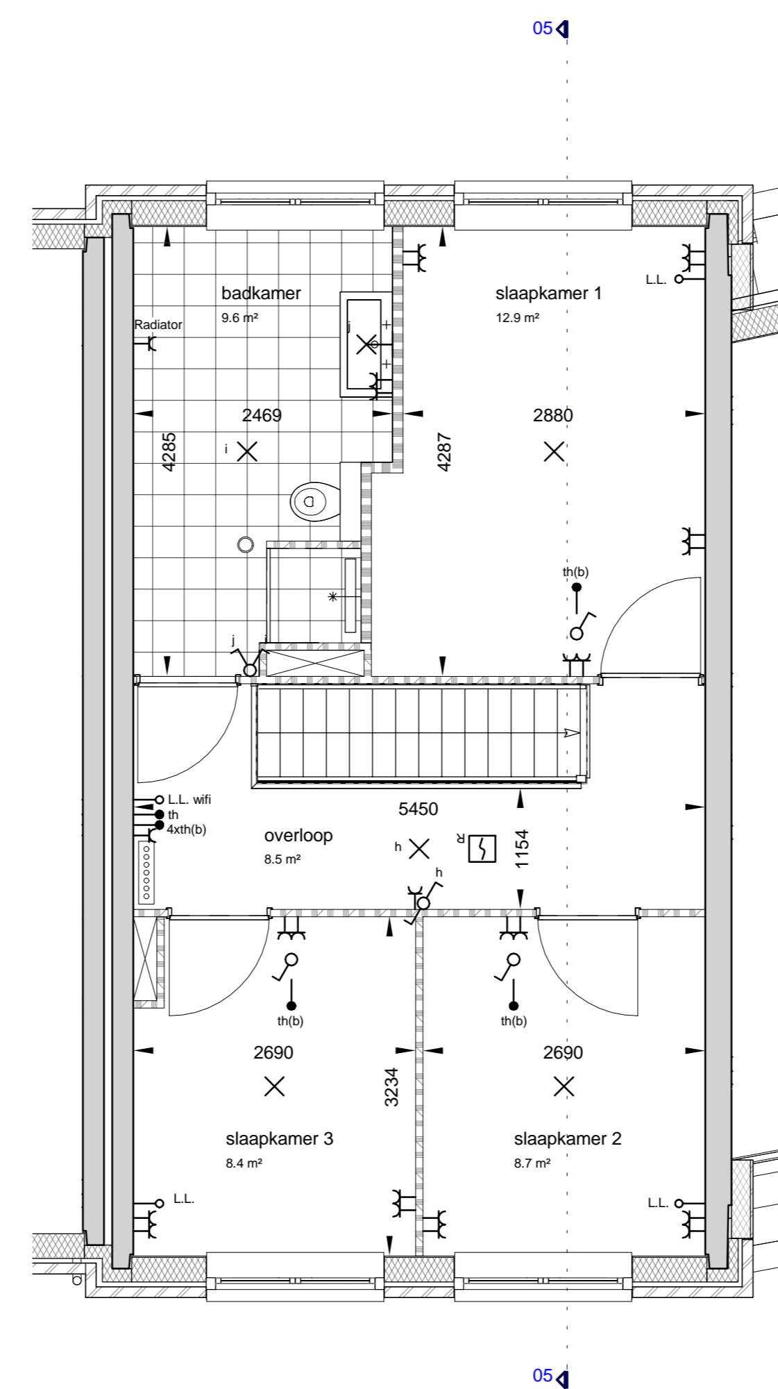
tweede verdieping
