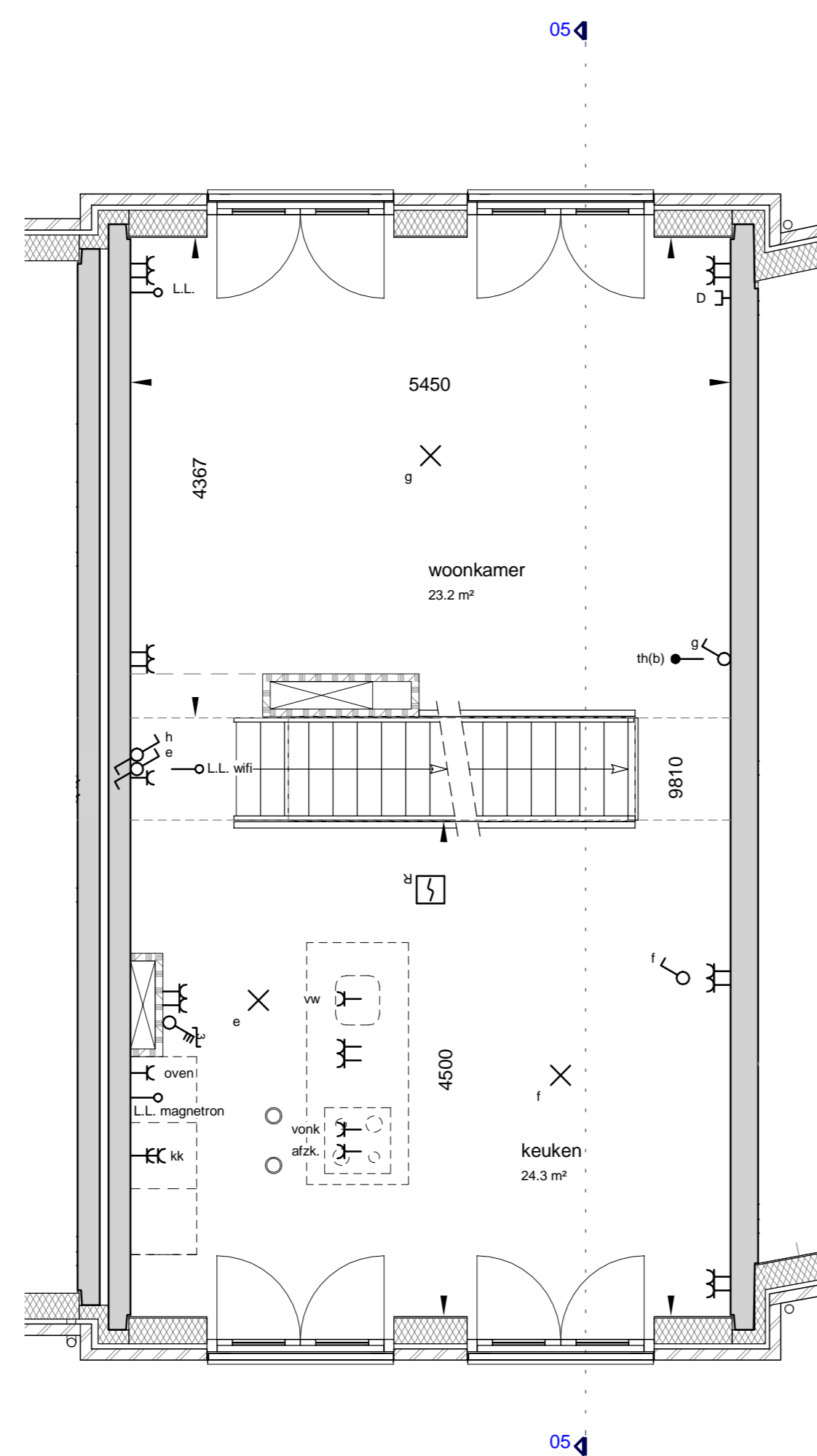
eerste verdieping
