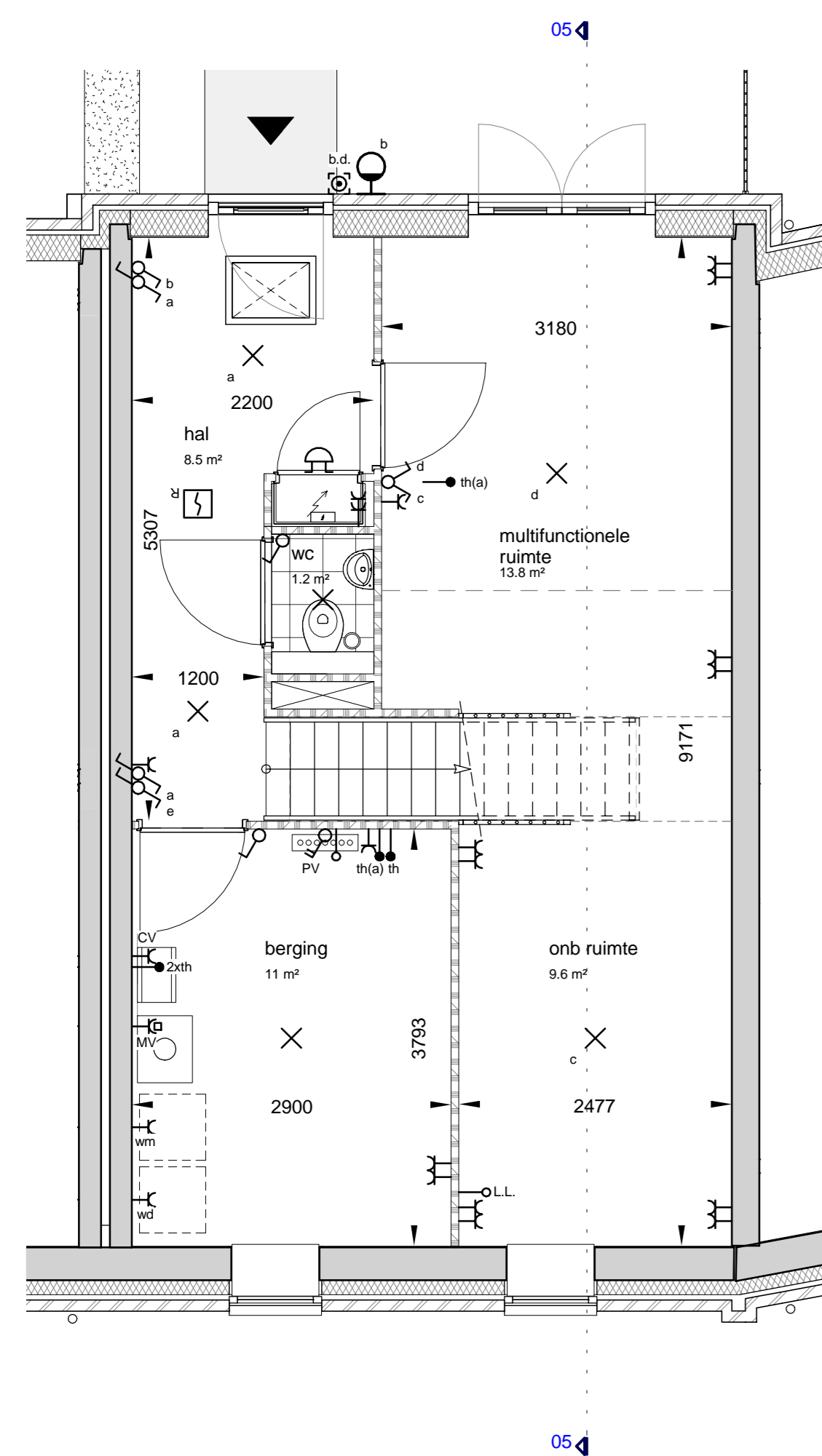
begane grond
