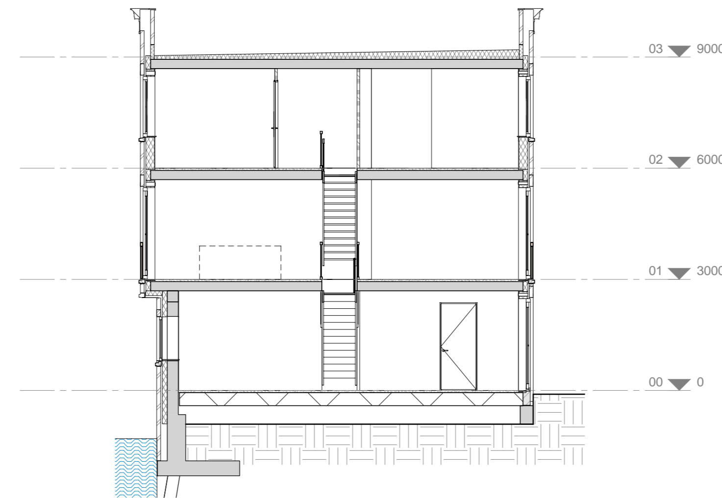
doorsnede
