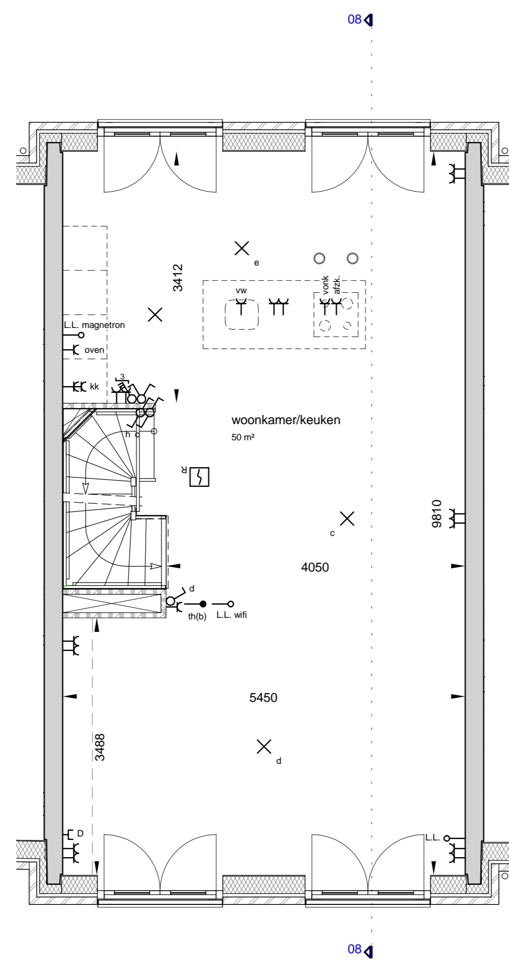
eerste verdieping
