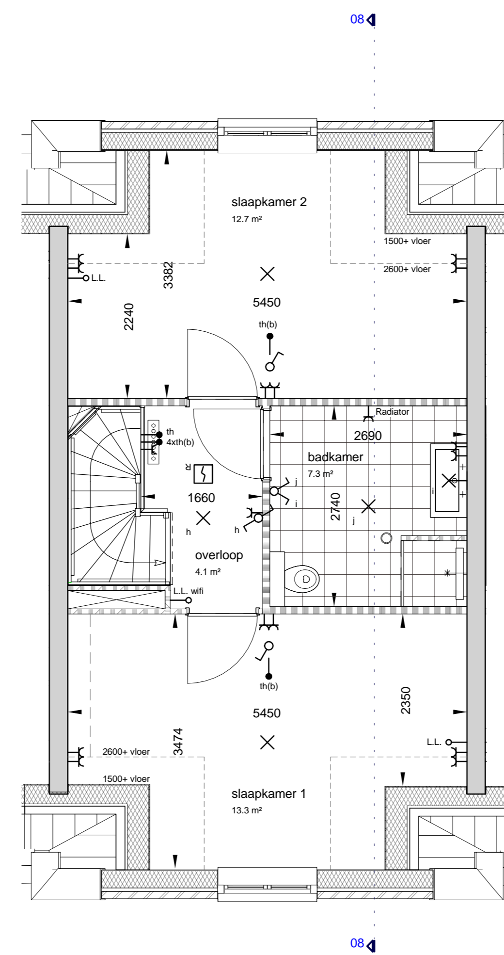
tweede verdieping
