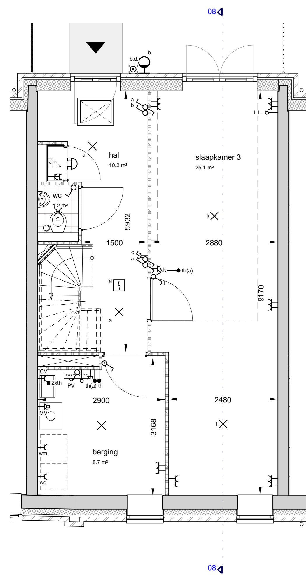
begane grond
