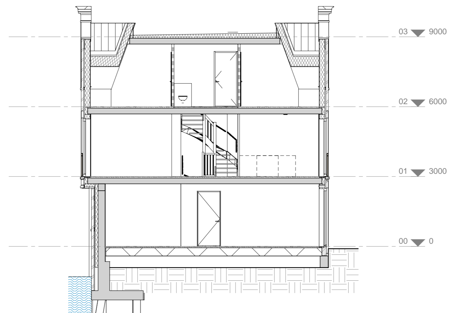
doorsnede
