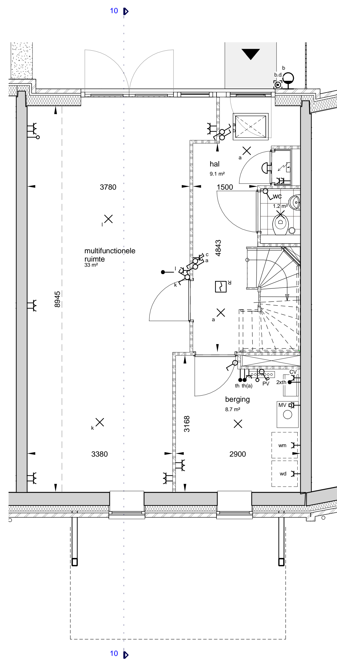
begane grond
