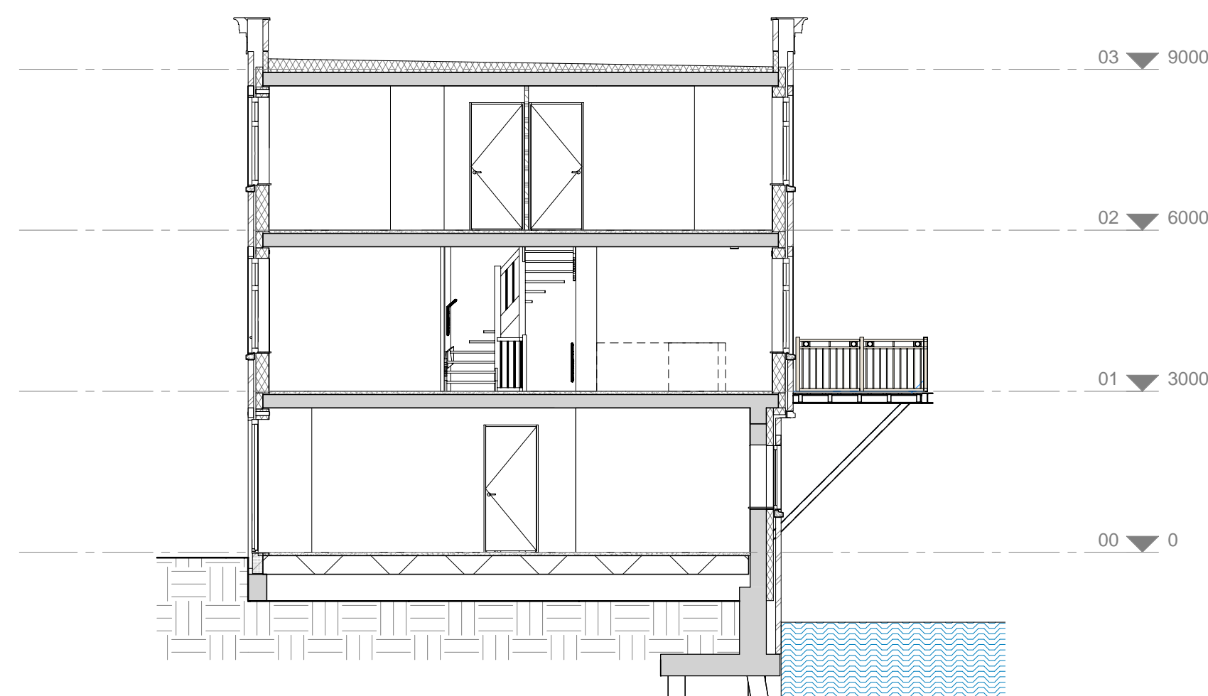
doorsnede
