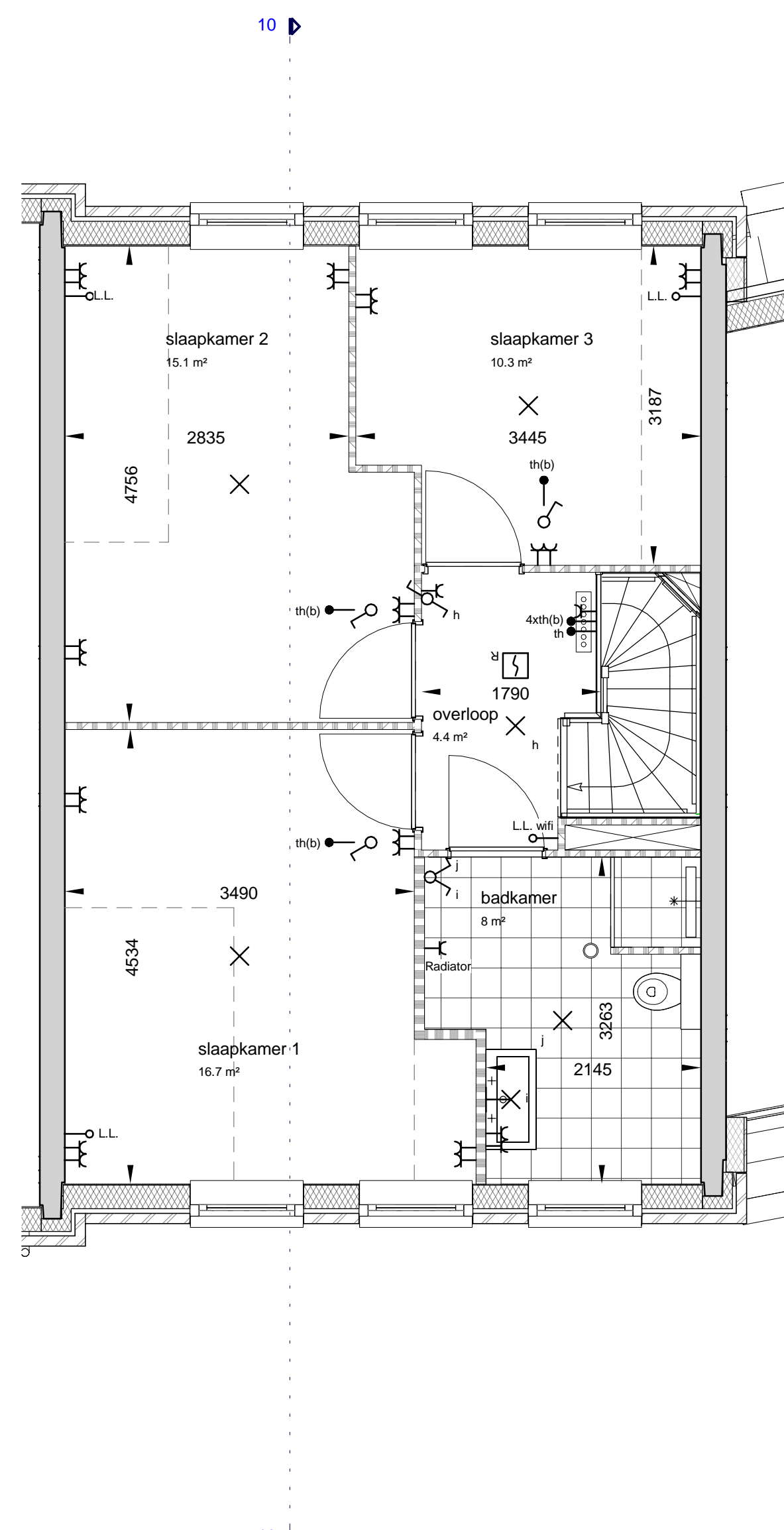
tweede verdieping
