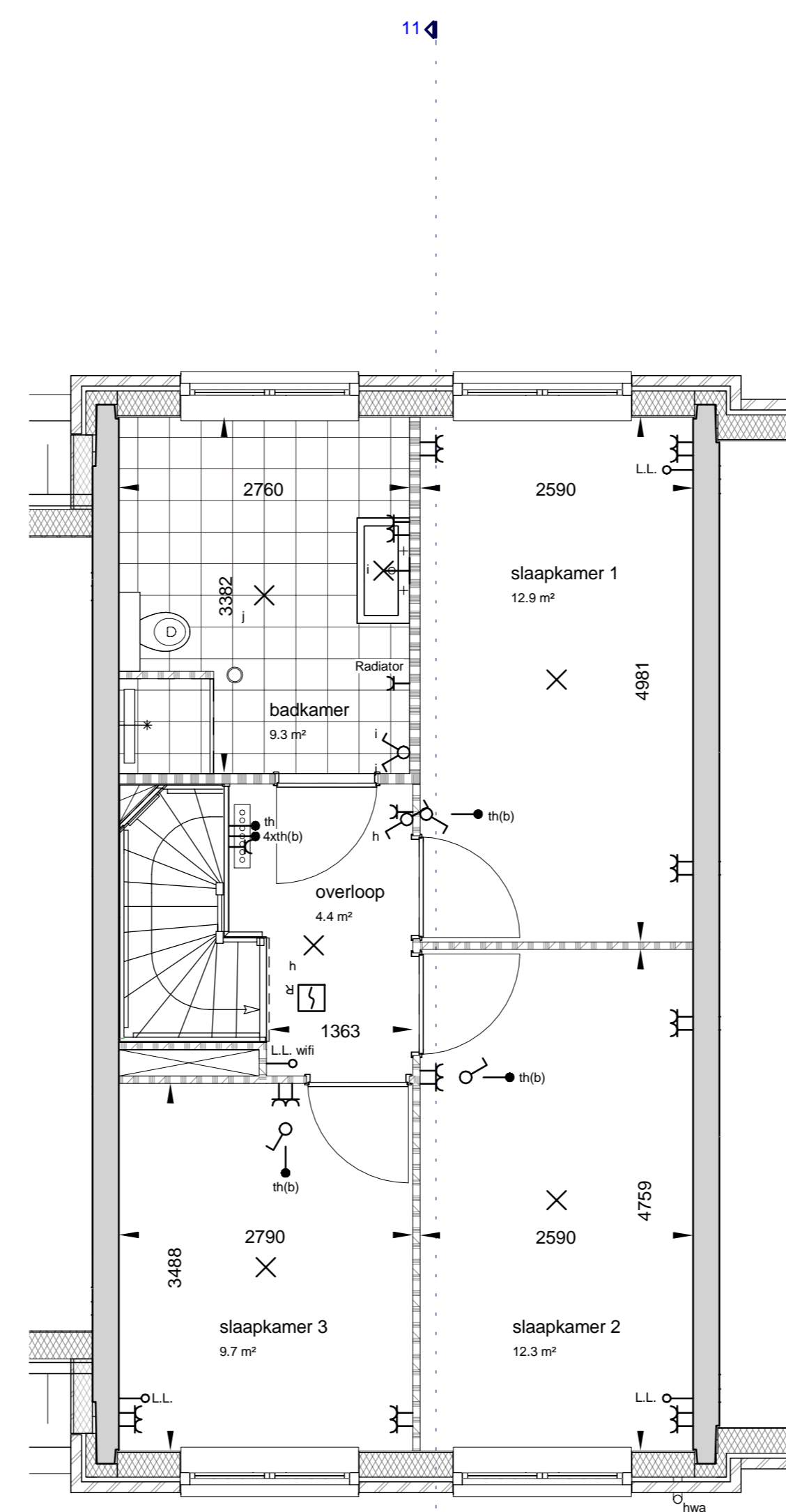
tweede verdieping
