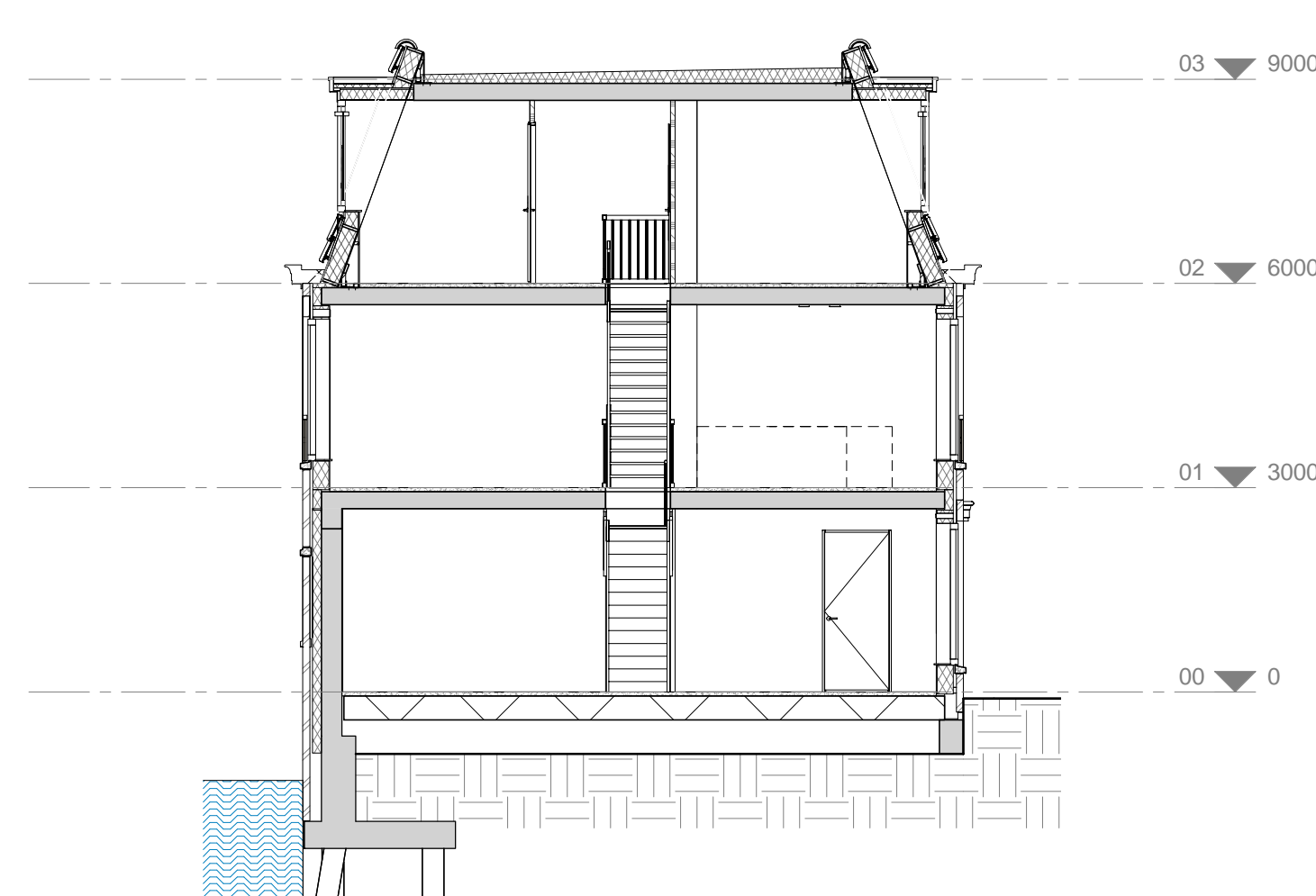
doorsnede
