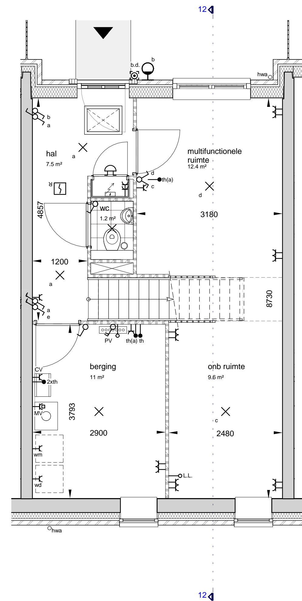
begane grond
