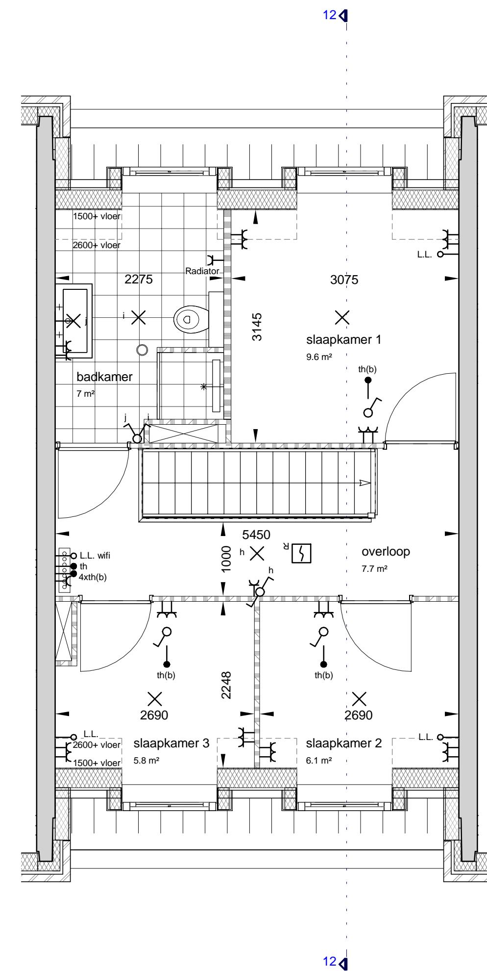
tweede verdieping
