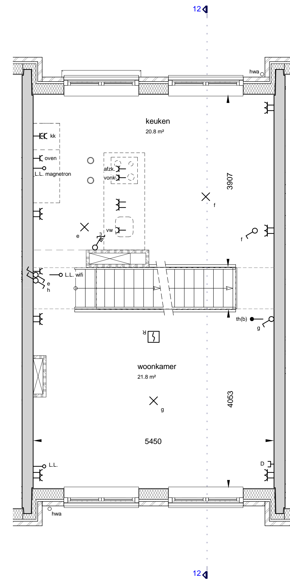
eerste verdieping
