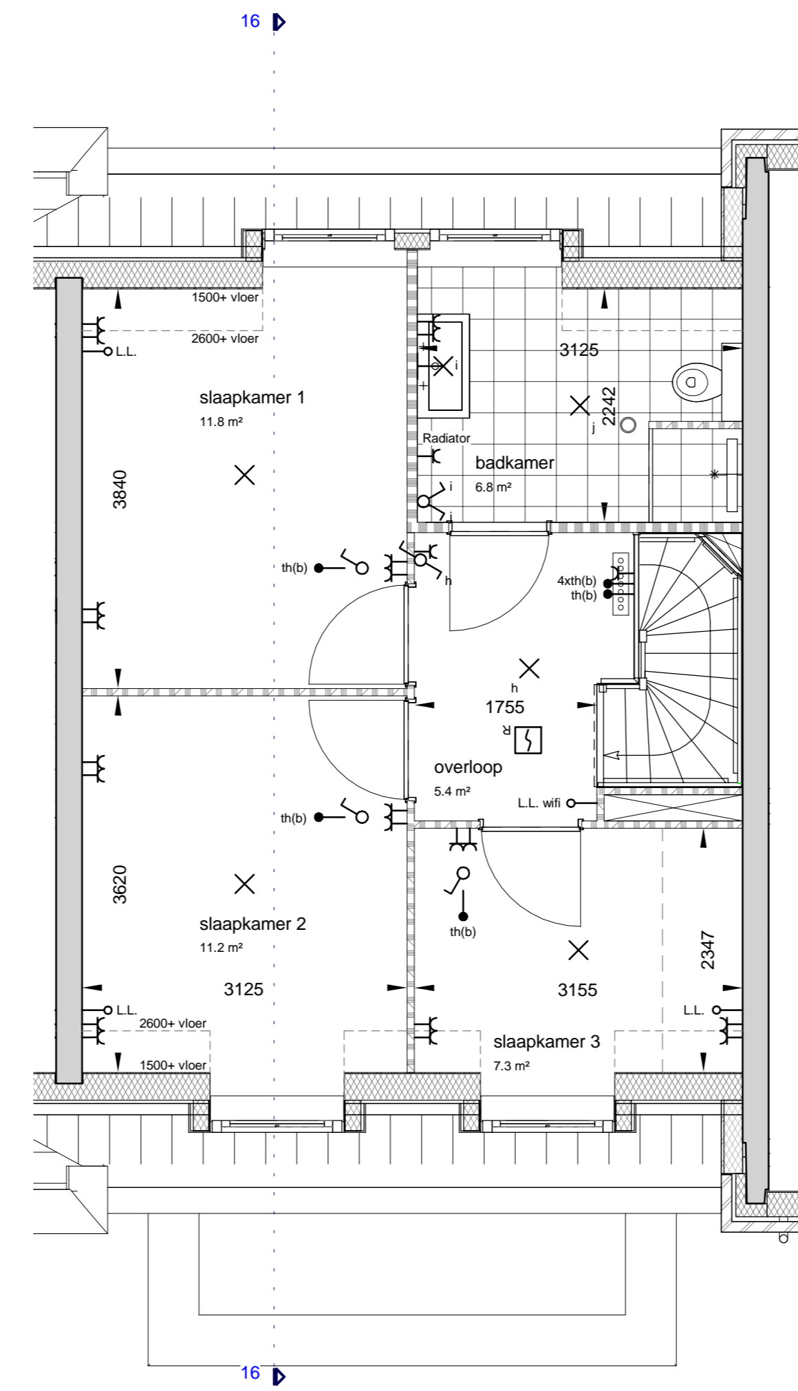
tweede verdieping
