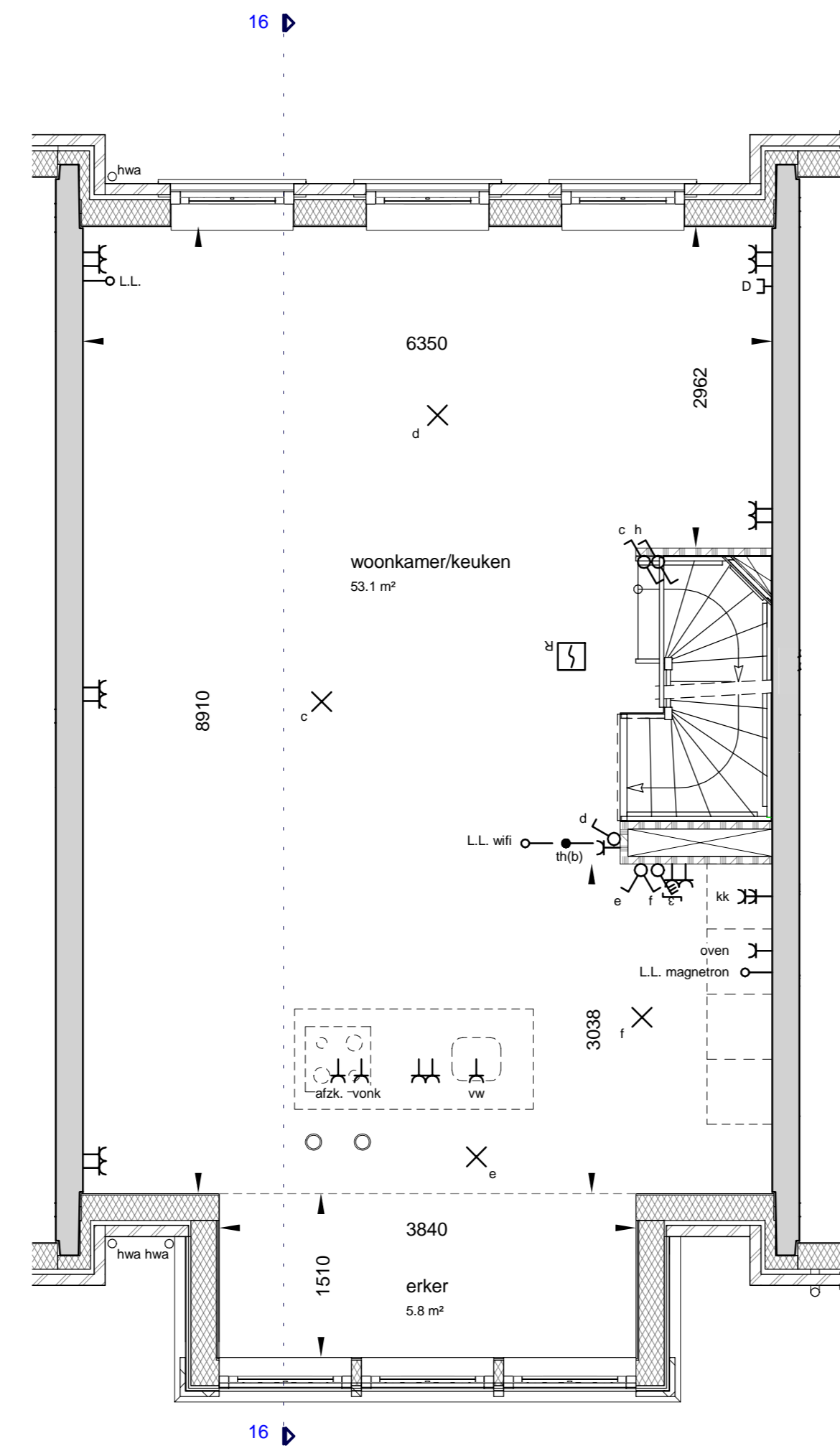
eerste verdieping
