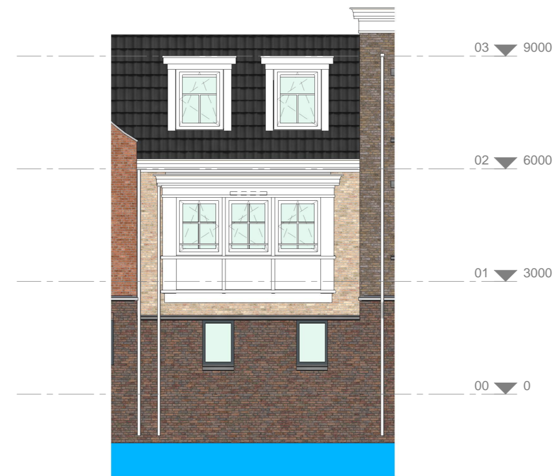
watergevel
