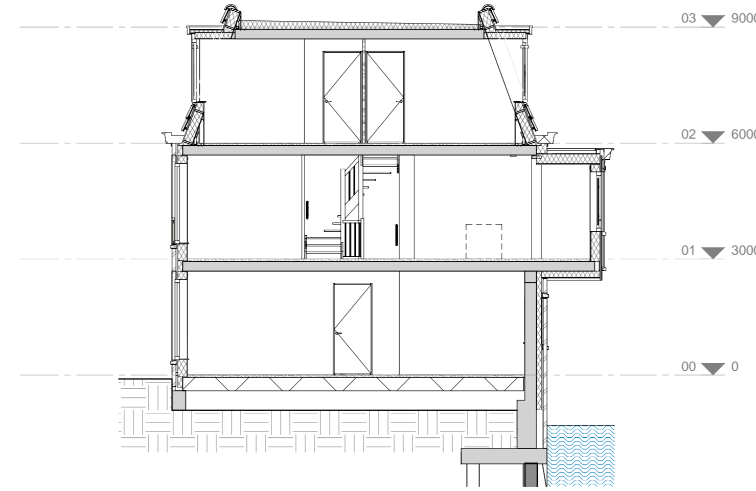
doorsnede
