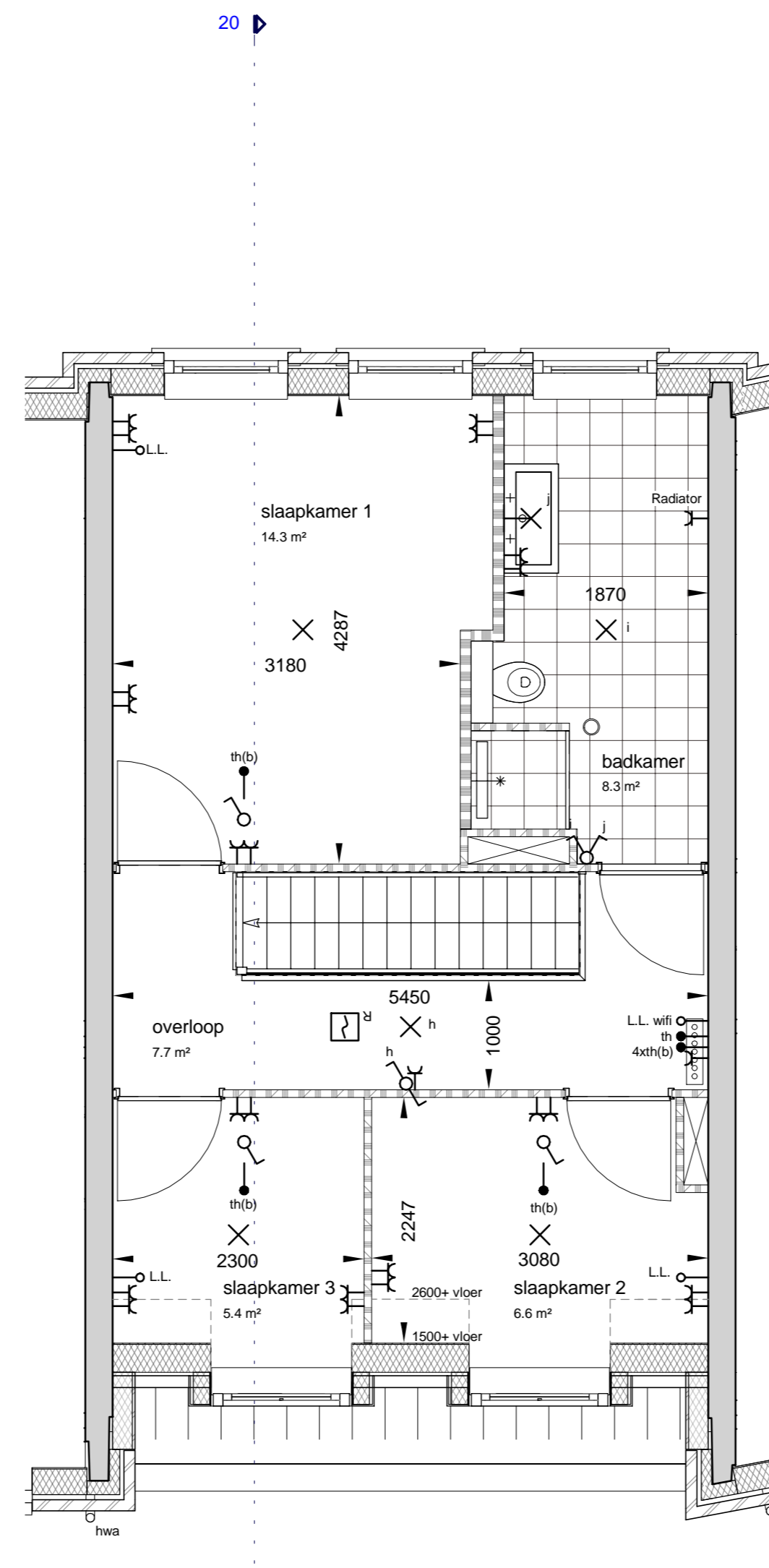
tweede verdieping
