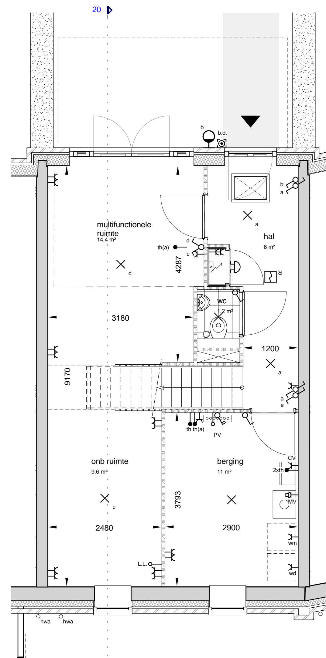
begane grond
