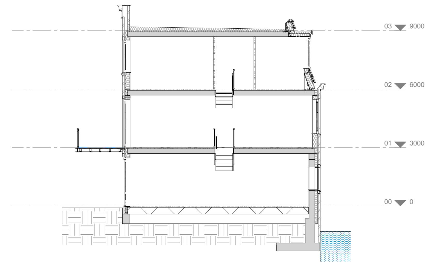
doorsnede
