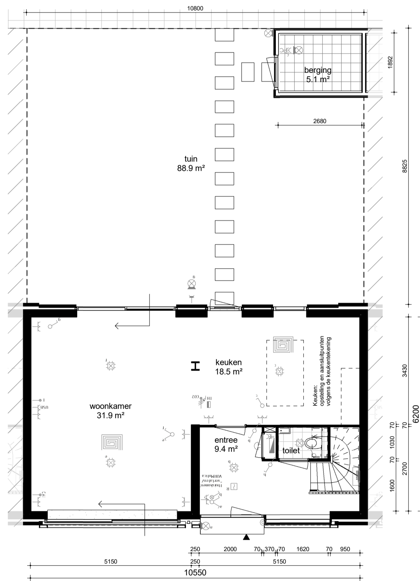
begane grond
