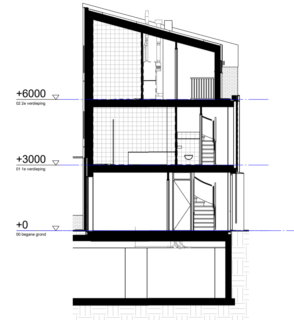
Doorsnede
