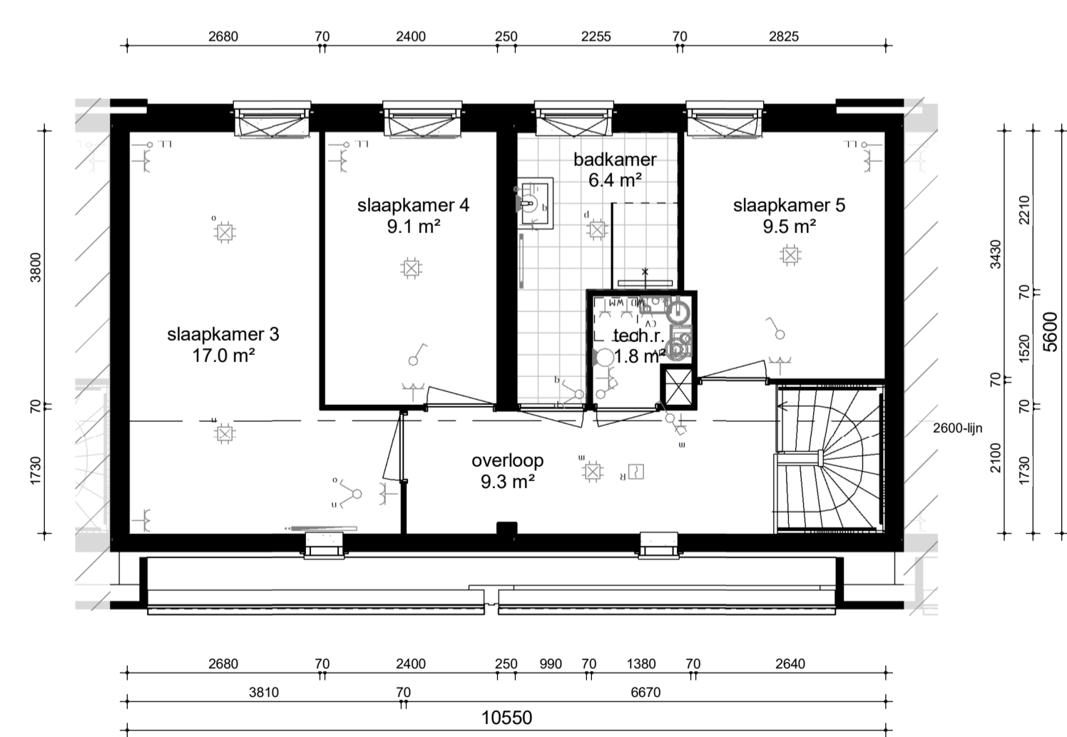
2e verdieping
