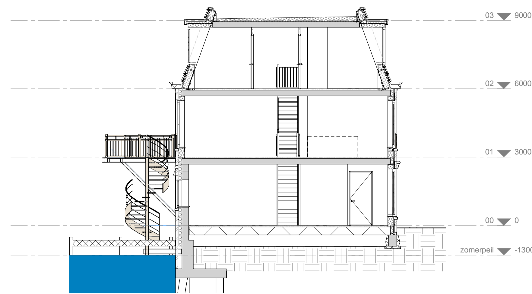
doorsnede
