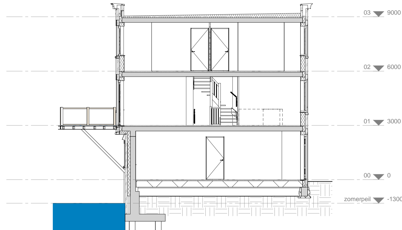
doorsnede
