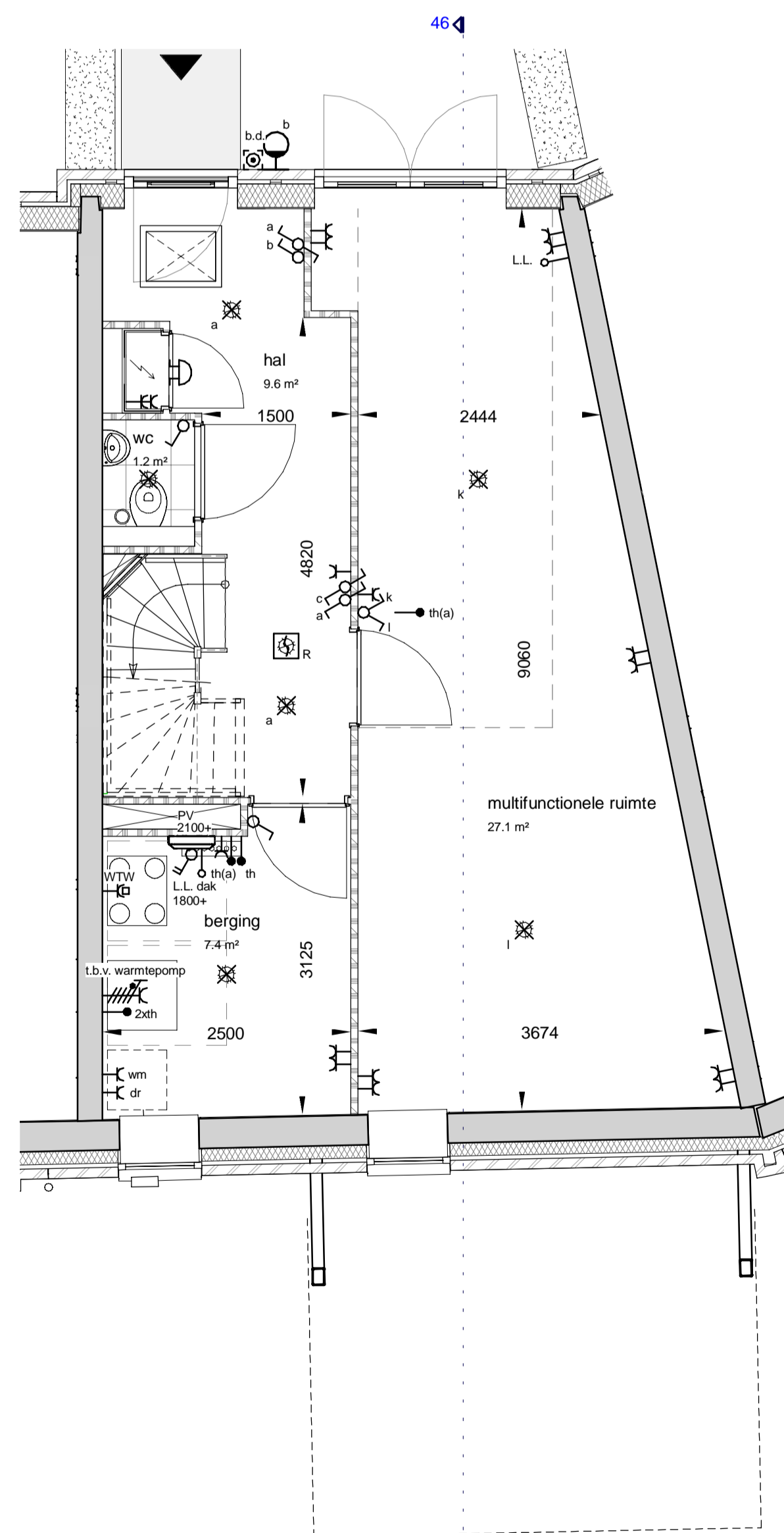
begane grond
