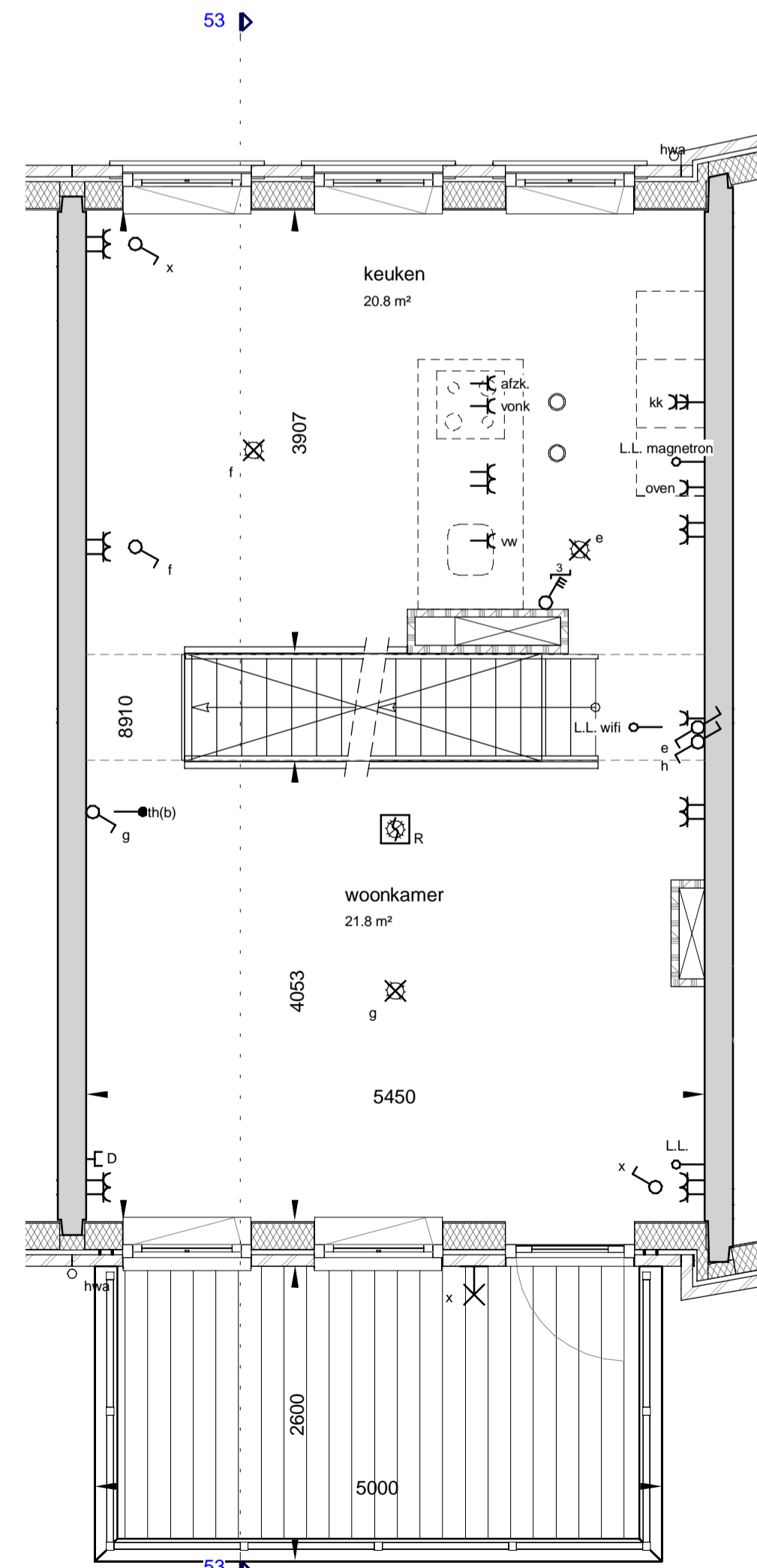
eerste verdieping
