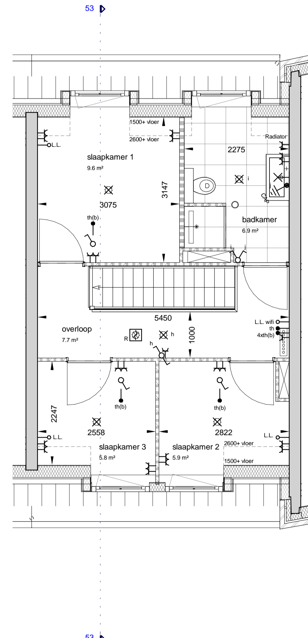
tweede verdieping
