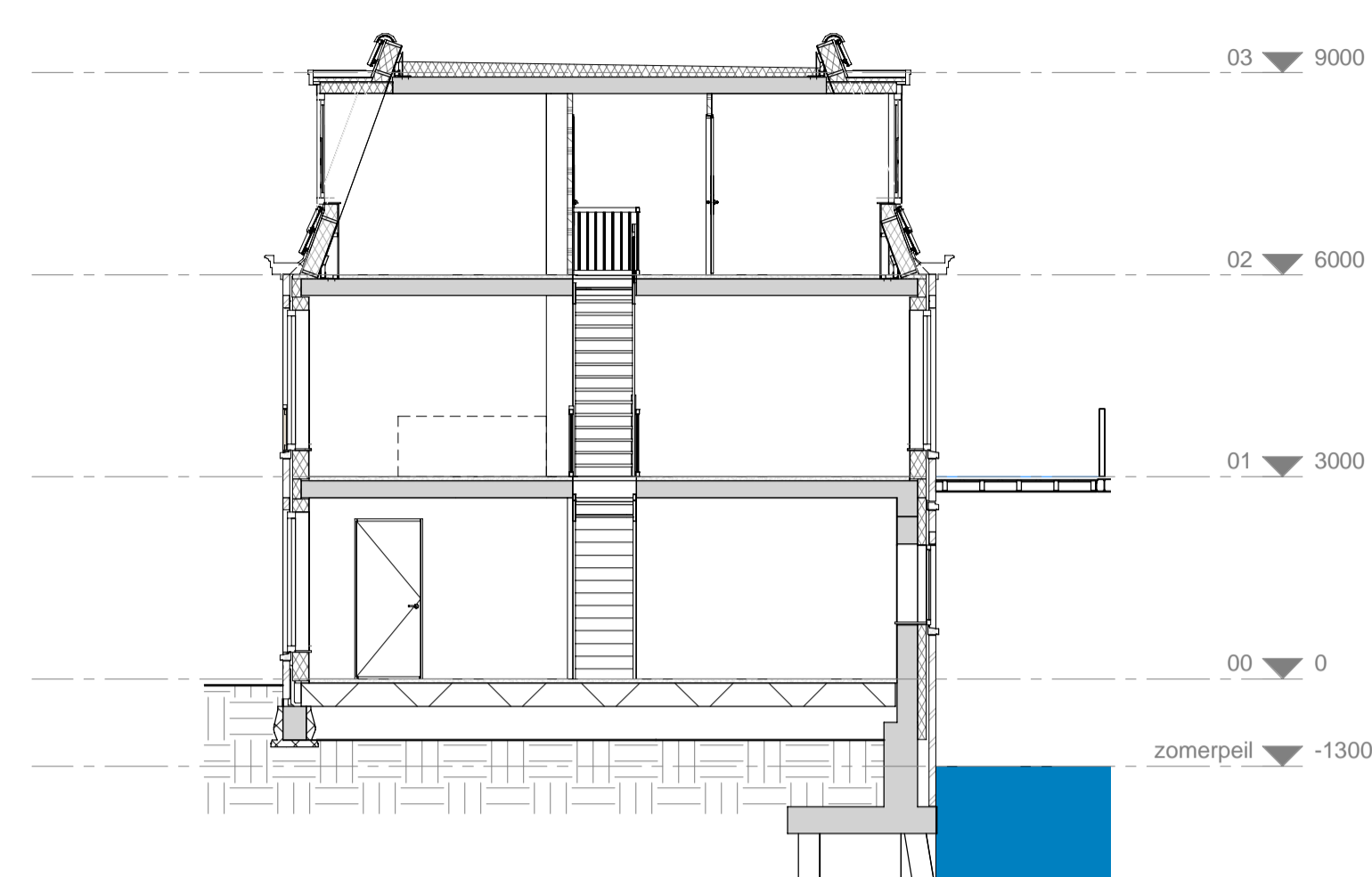
doorsnede
