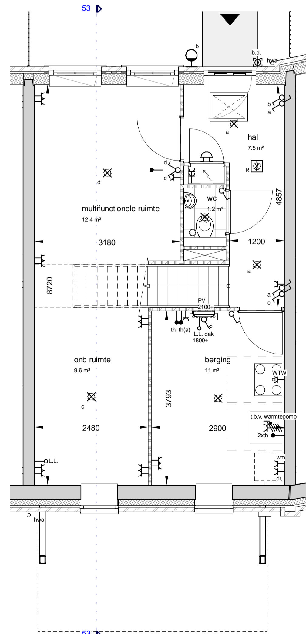
begane grond
