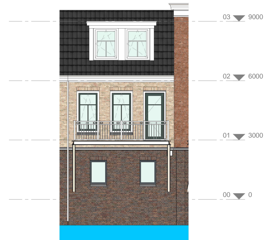
watergevel
