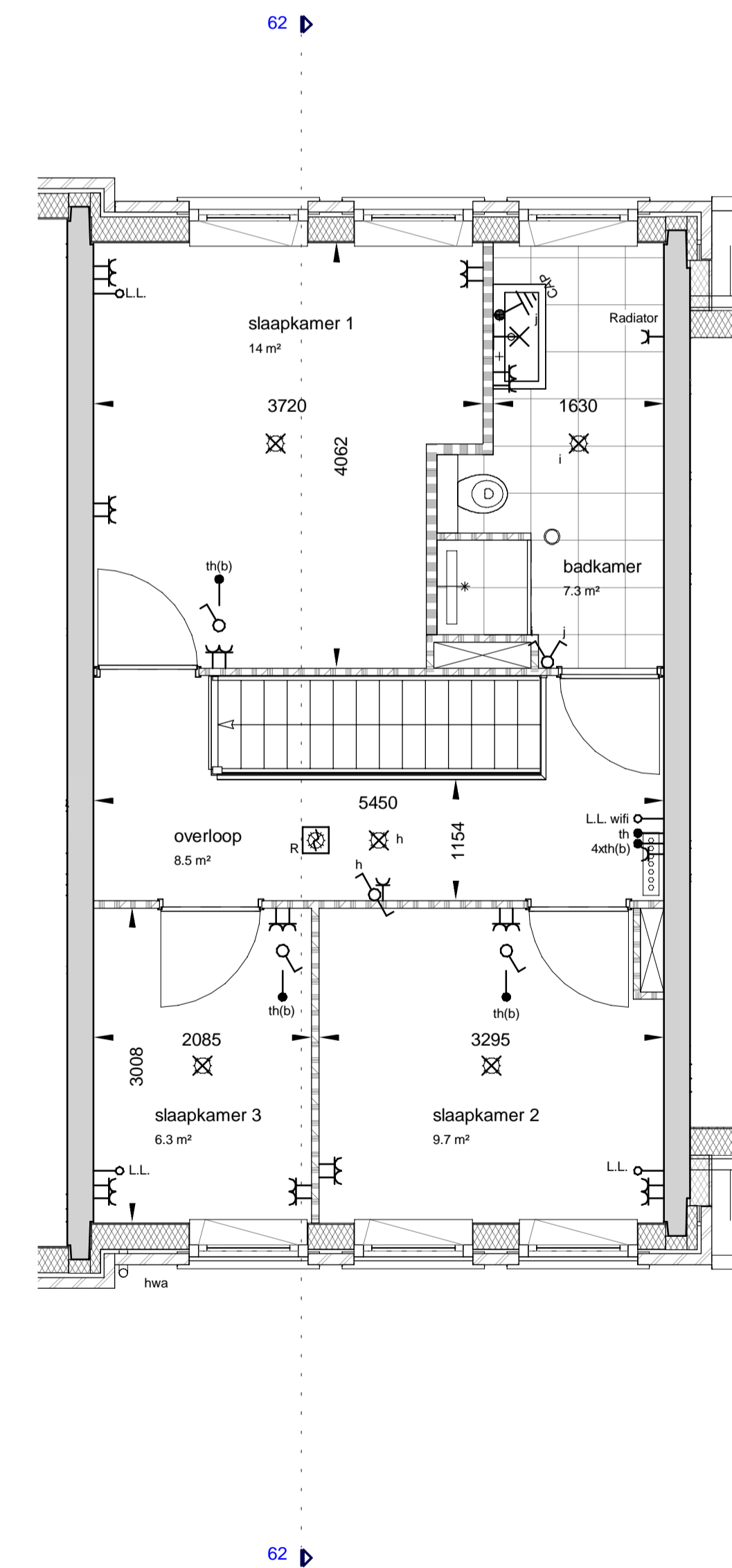
tweede verdieping
