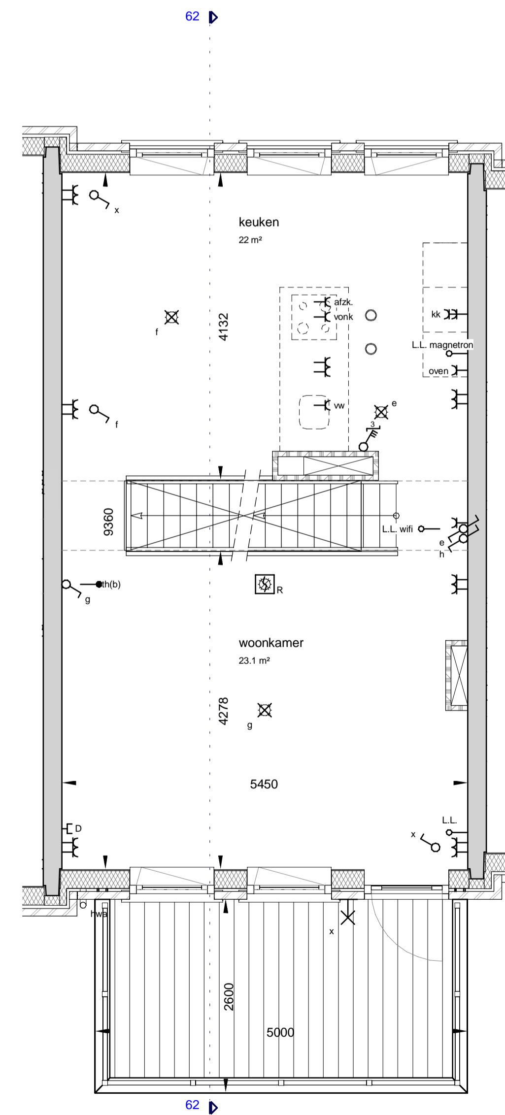
eerste verdieping
