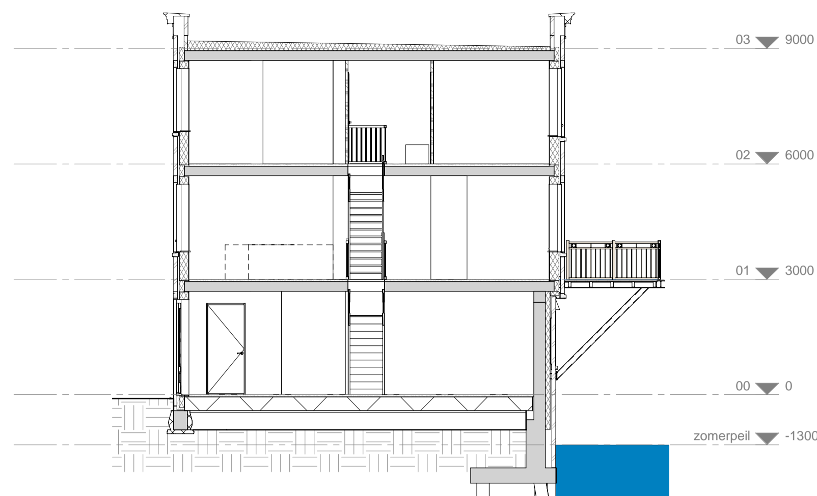
doorsnede
