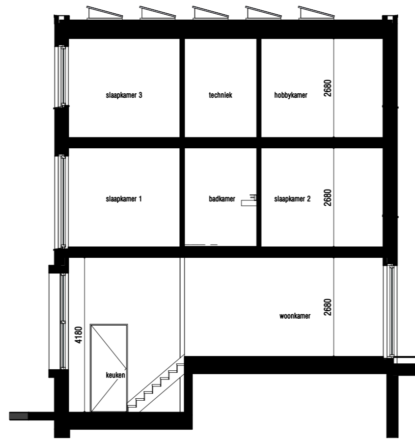
doorsnede 1:100
