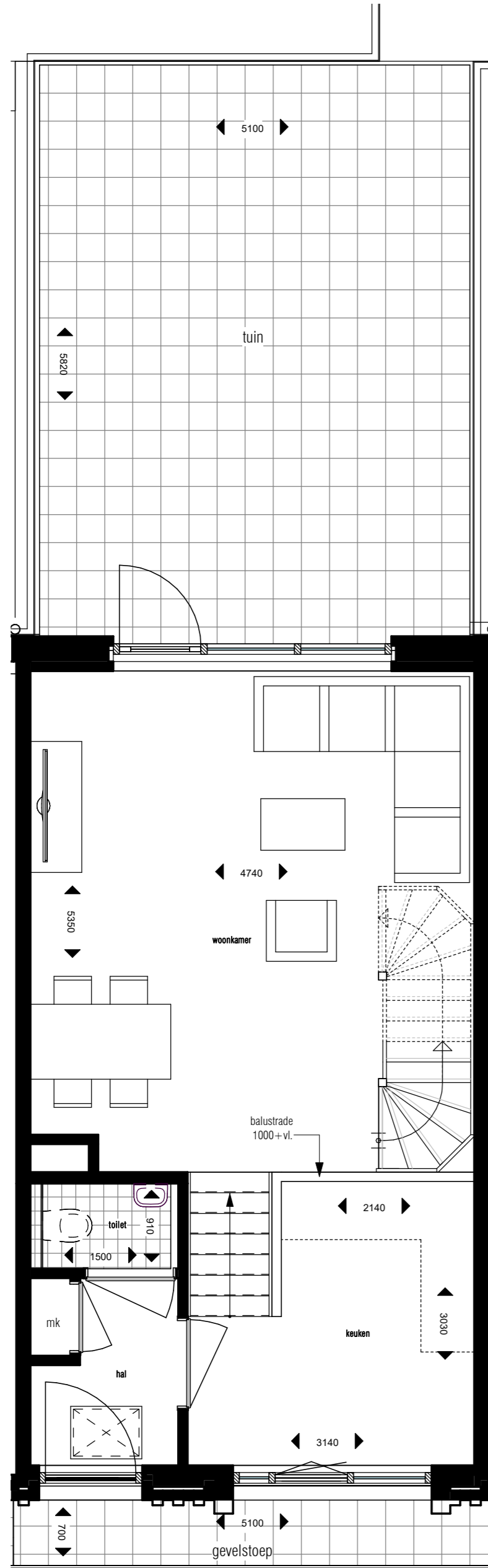
Bwnr:44 begane grond 1:50
