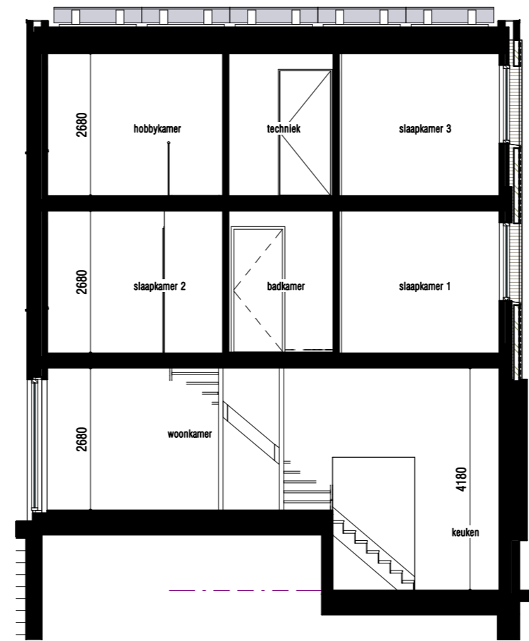
doorsnede 1:100
