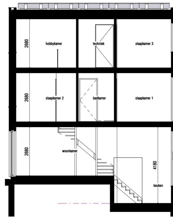
doorsnede 1:100
