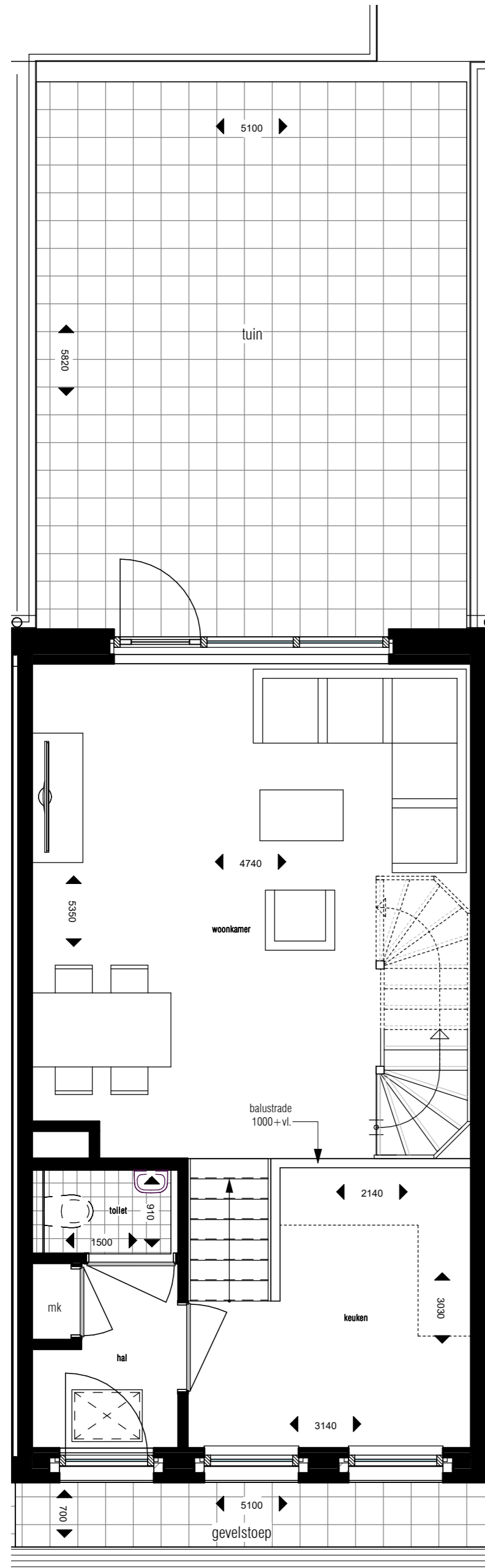
Bwnr:42 begane grond 1:50
