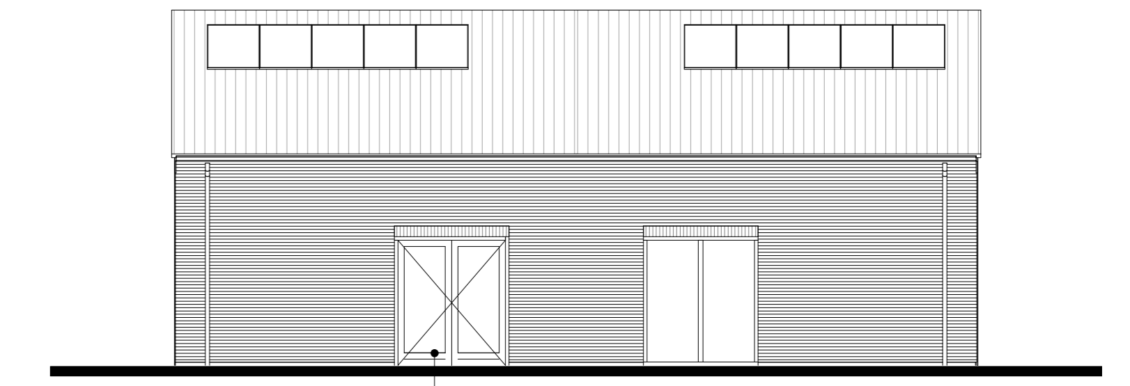
Zuidgevel SCHAAL 1 : 100
