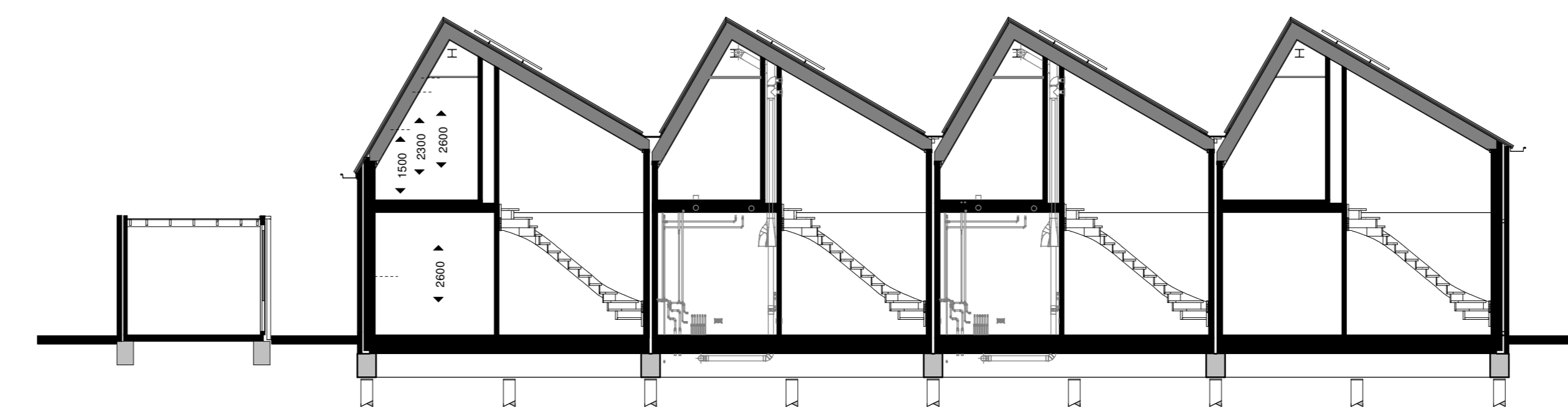
Doorsnede SCHAAL 1 : 100
