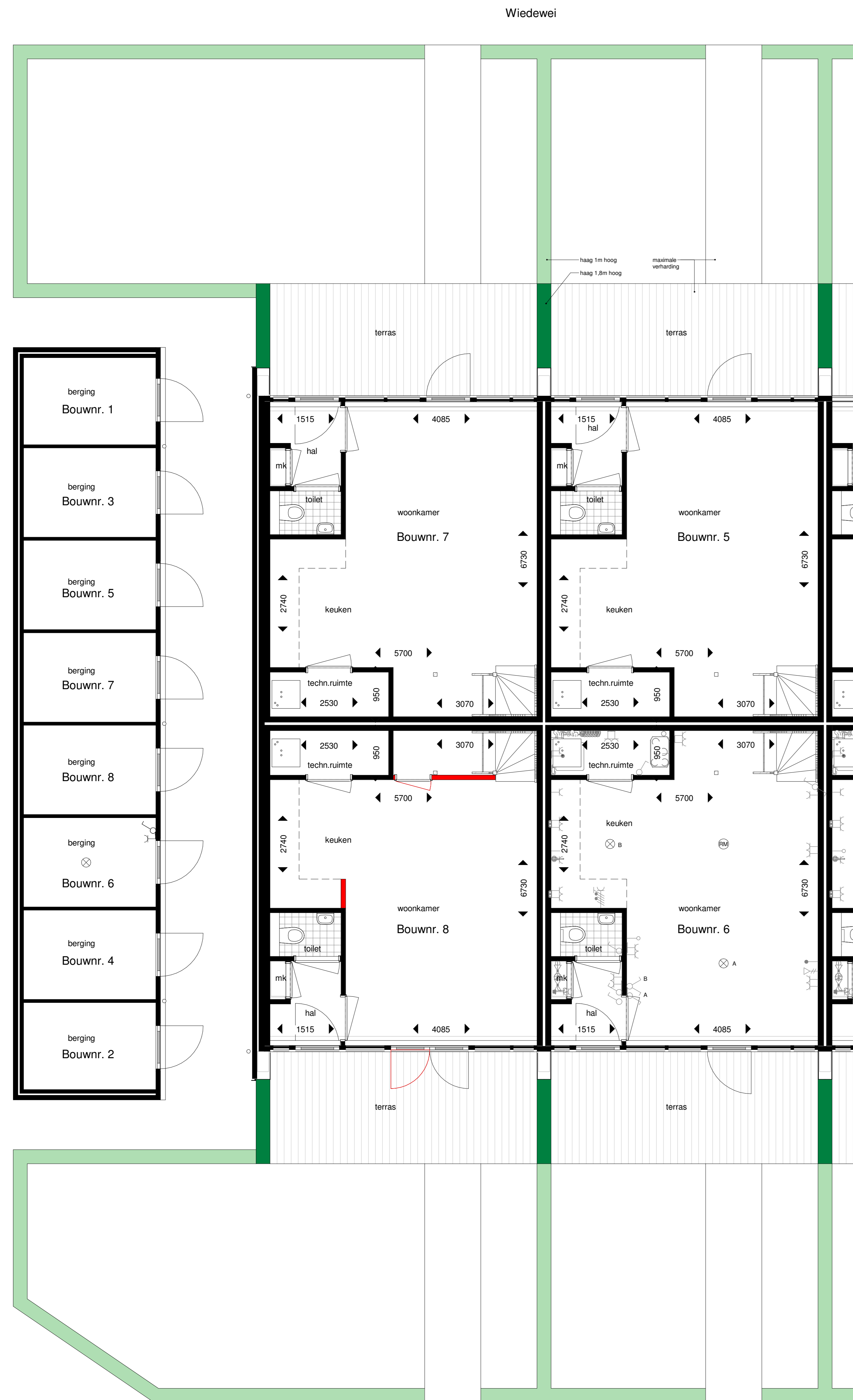
Begane grond SCHAAL 1 : 50
