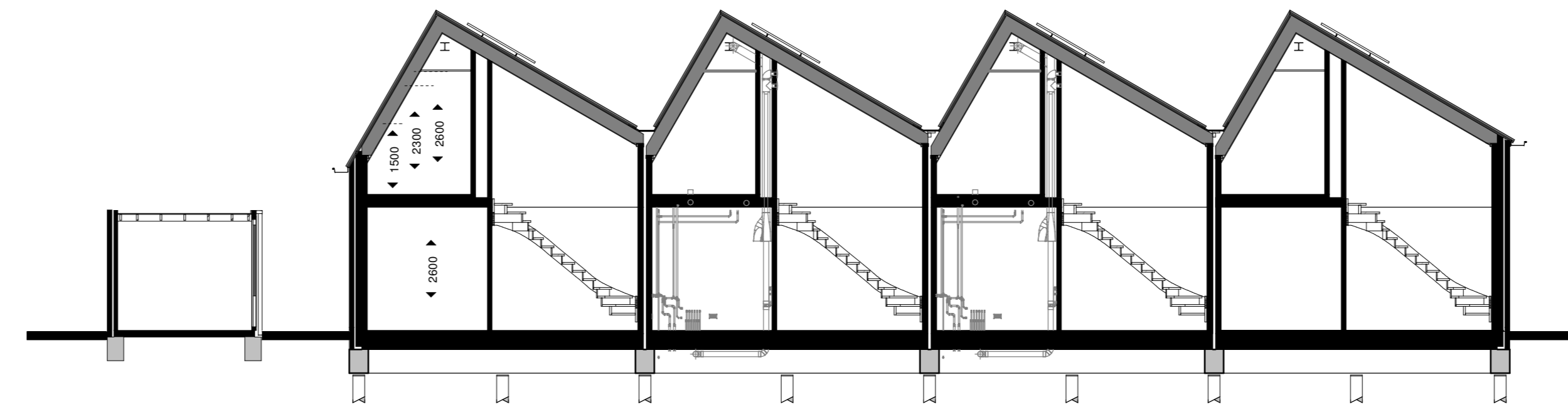
Doorsnede SCHAAL 1 : 100
