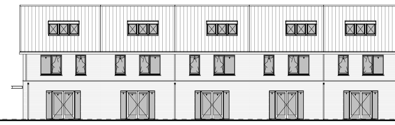
achtergevel Schaal: 1 : 200
