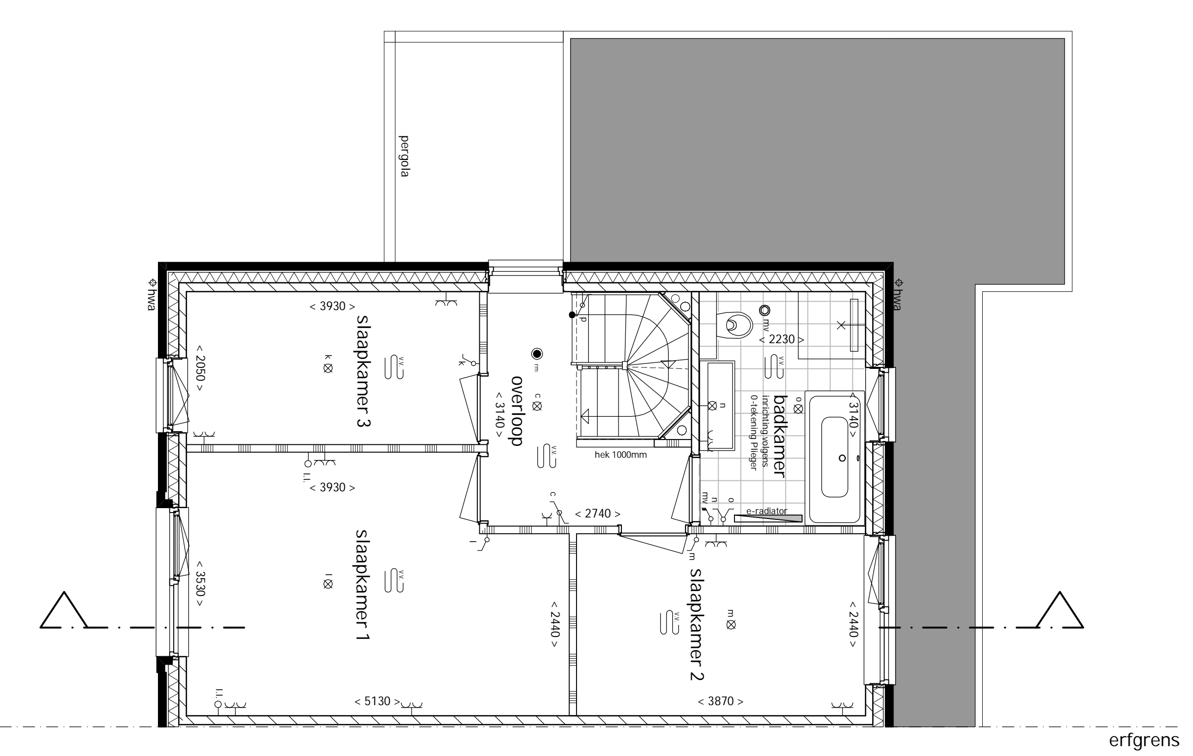
1e verdieping
