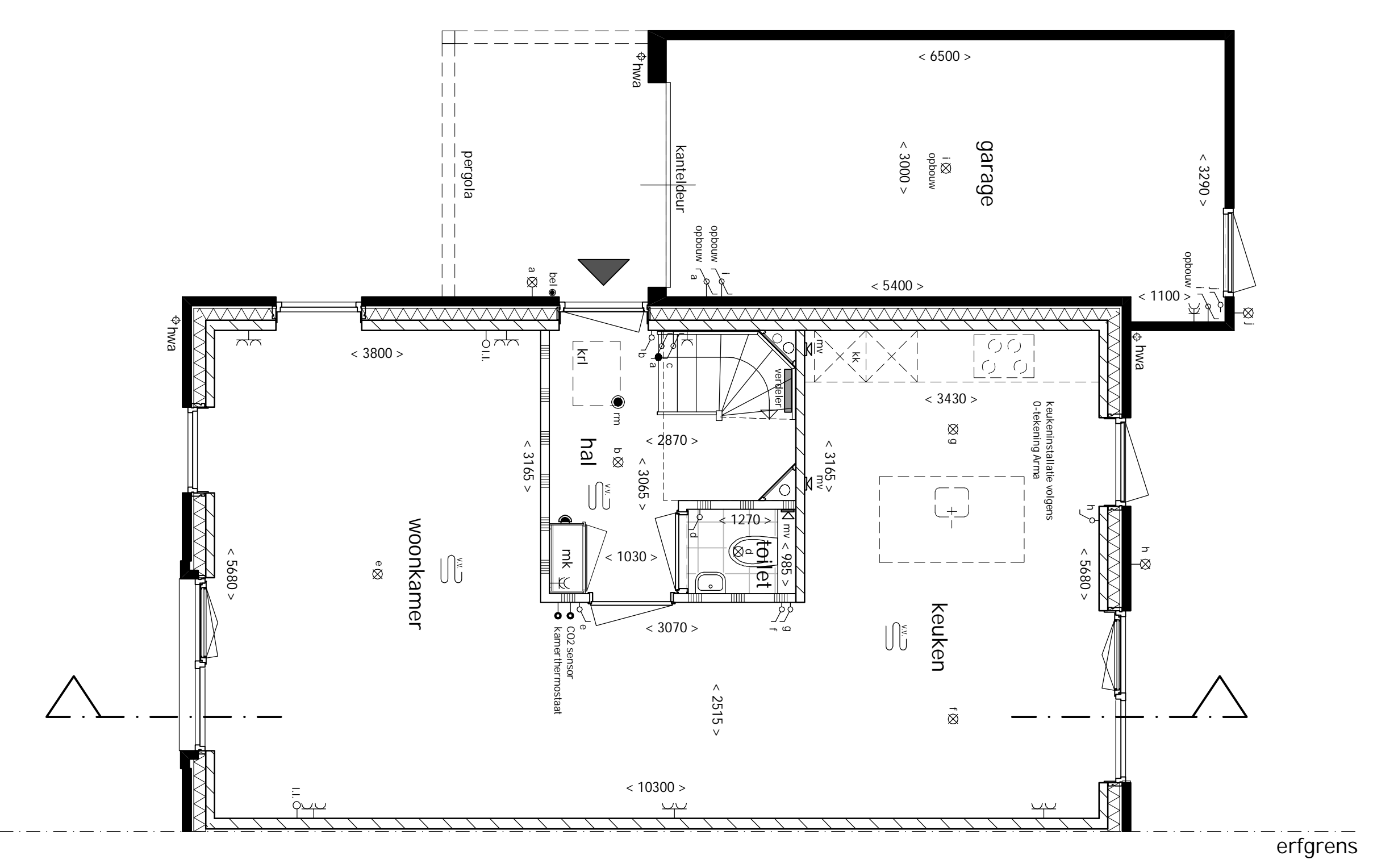
begane grond
