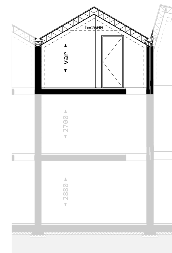
dwarsdoorsnede
