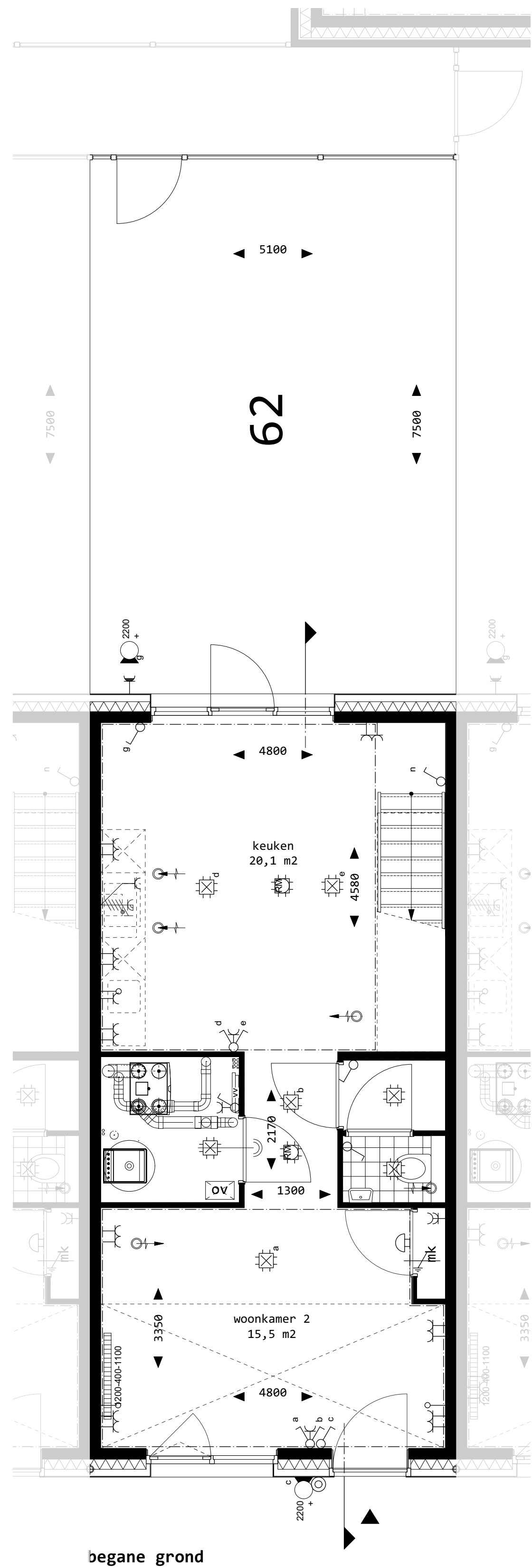
begane grond
