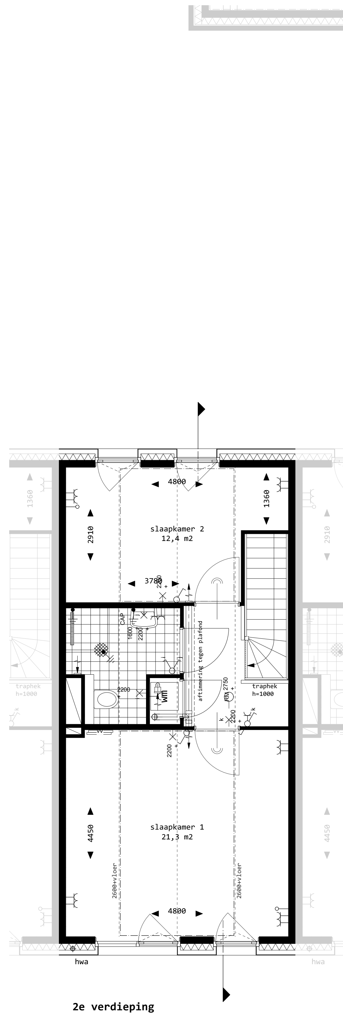
2e verdieping
