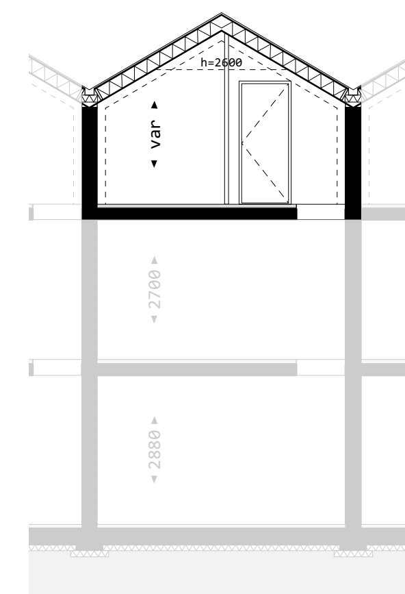
dwarsdoorsnede
