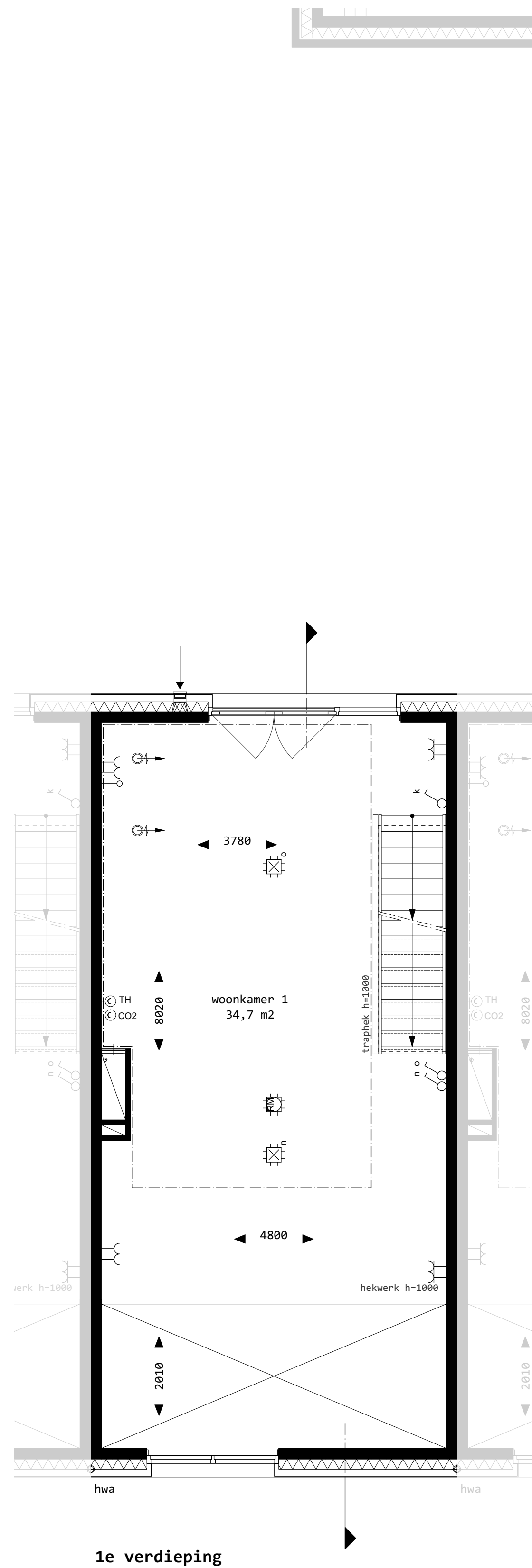
1e verdieping
