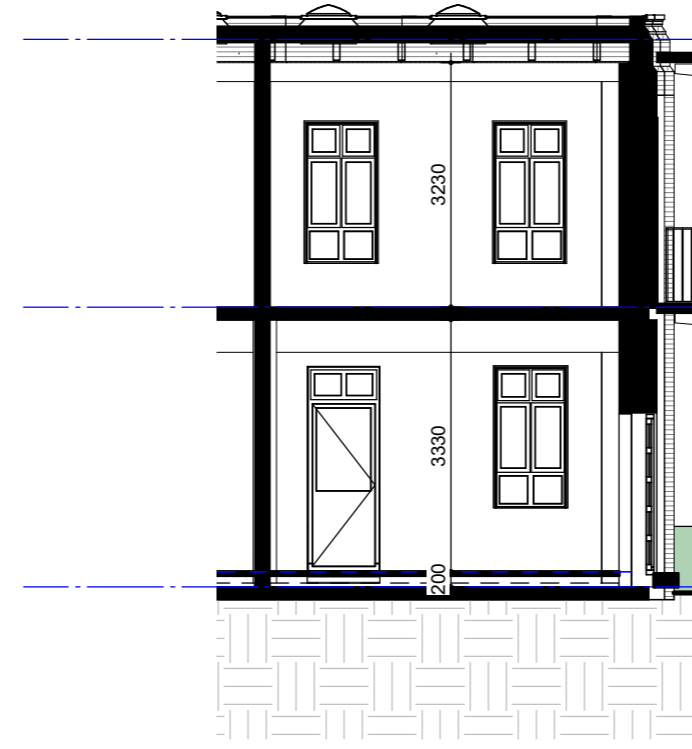
doorsnede A-A
