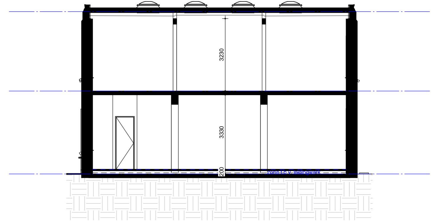
doorsnede B-B
