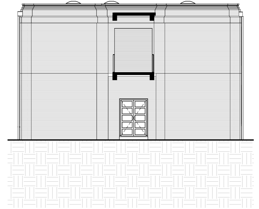
rechter zijgevel
