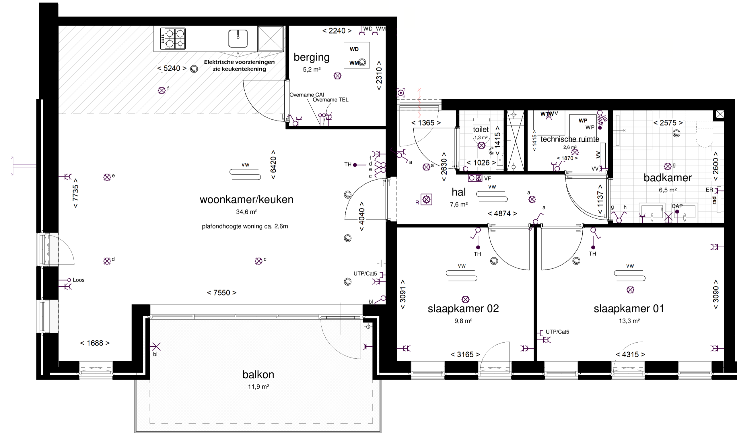
1:50 PLATTEGROND
