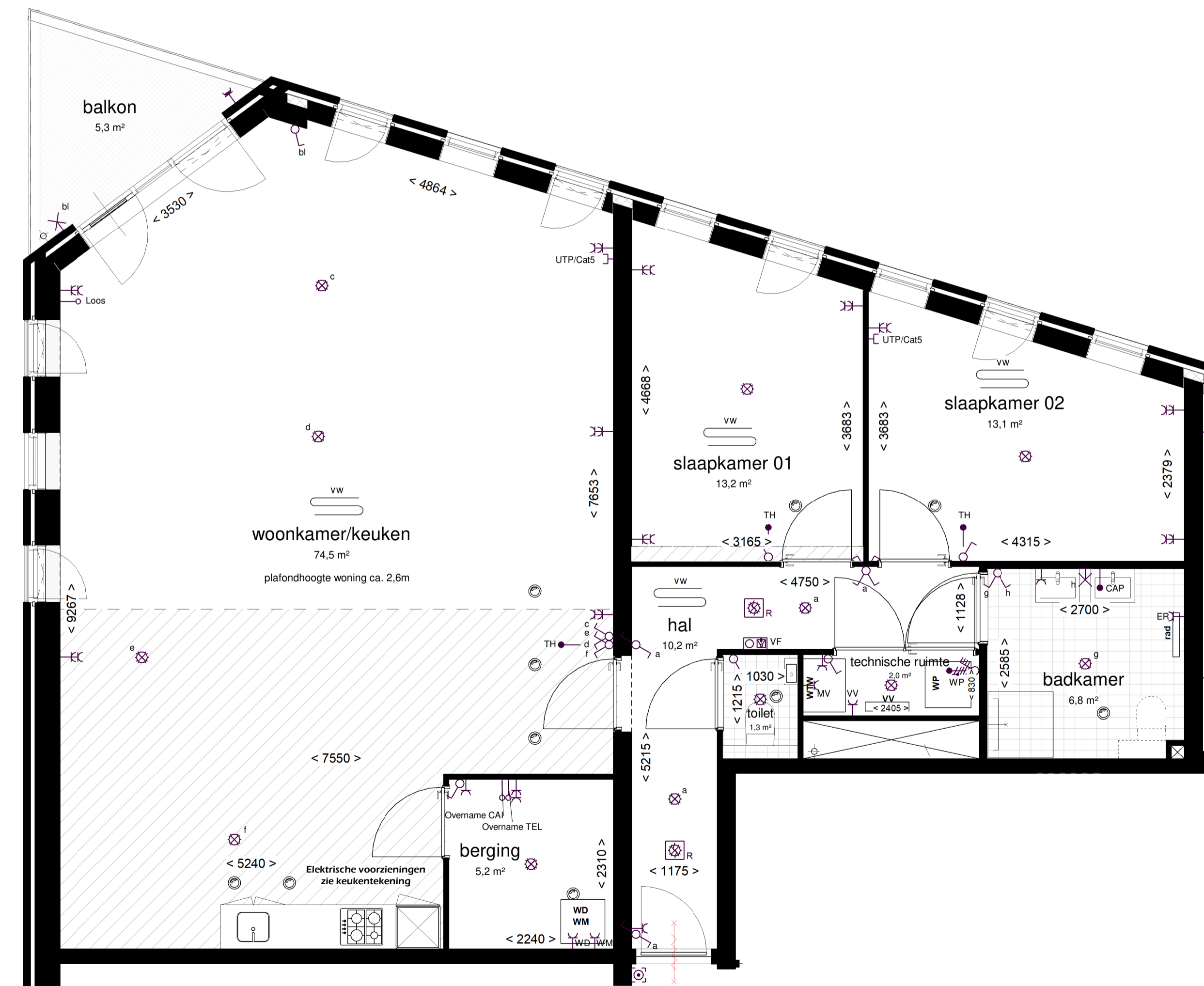
1:50 PLATTEGROND
