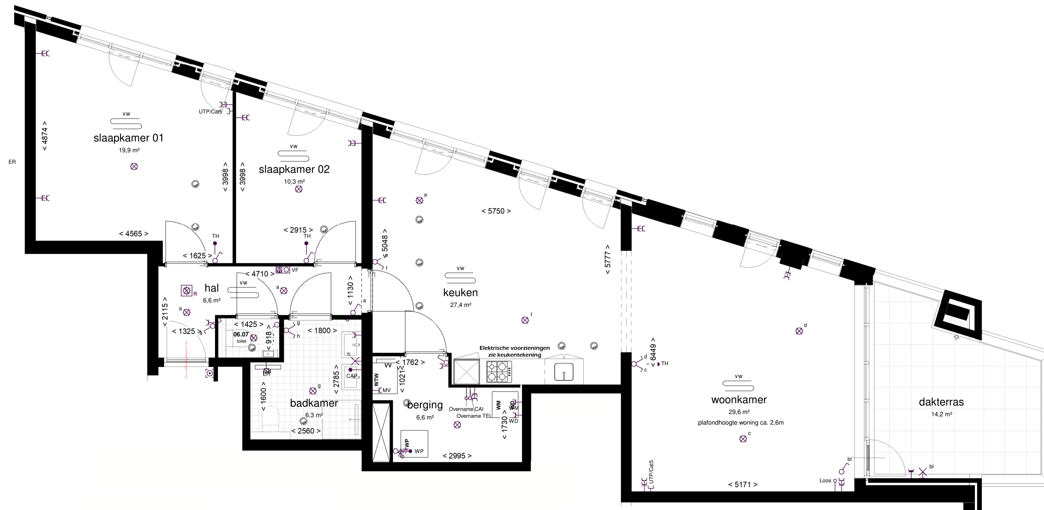
1 : 50 PLATTEGROND
