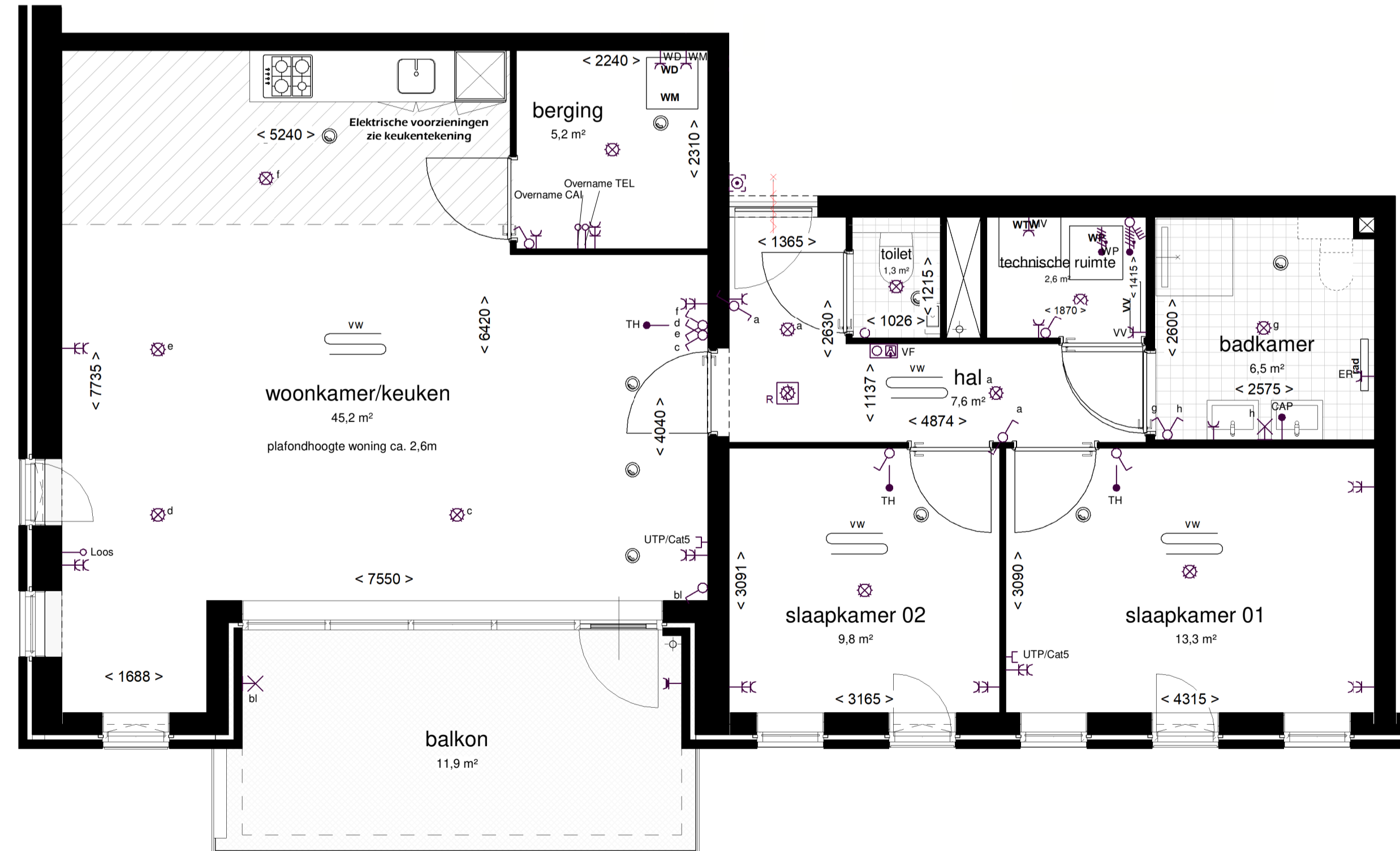
1:50 PLATTEGROND
