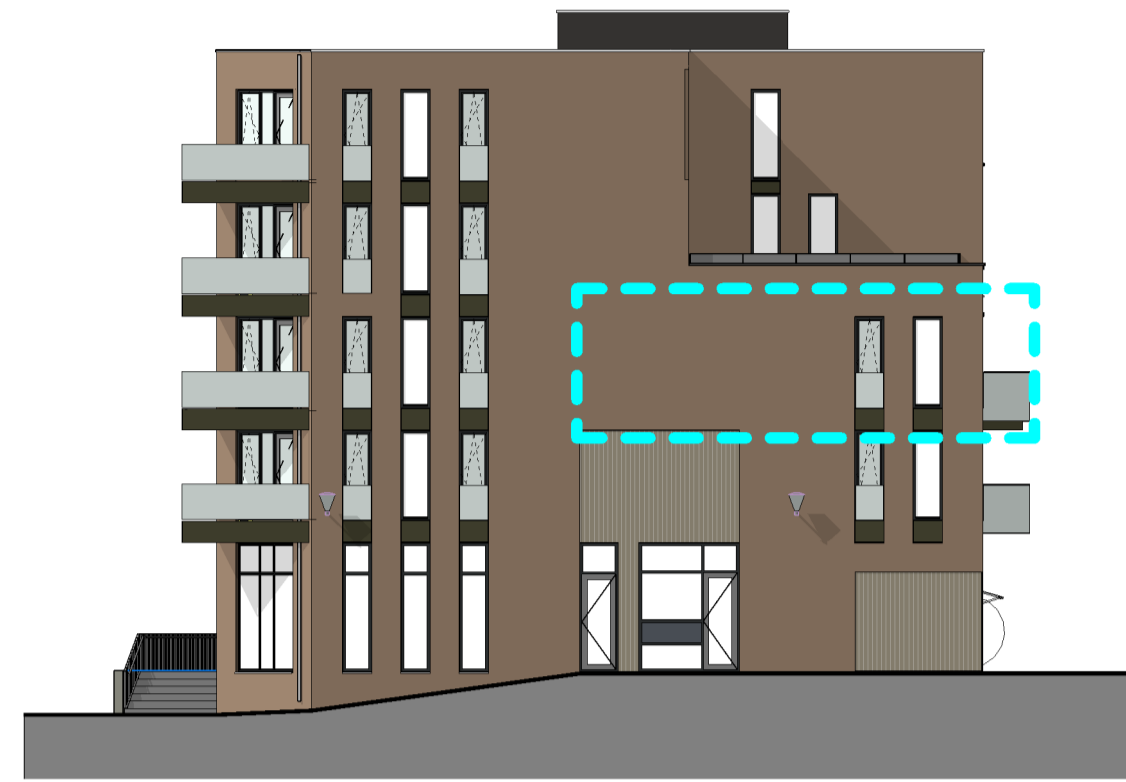
1:200 gevelaanzicht West
