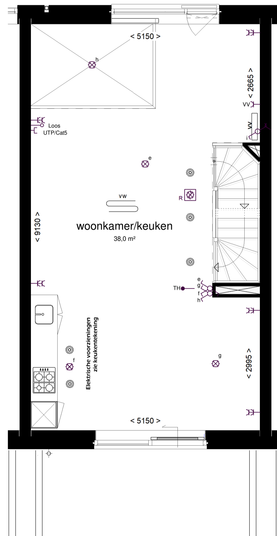
1:50 1e VERDIEPING
