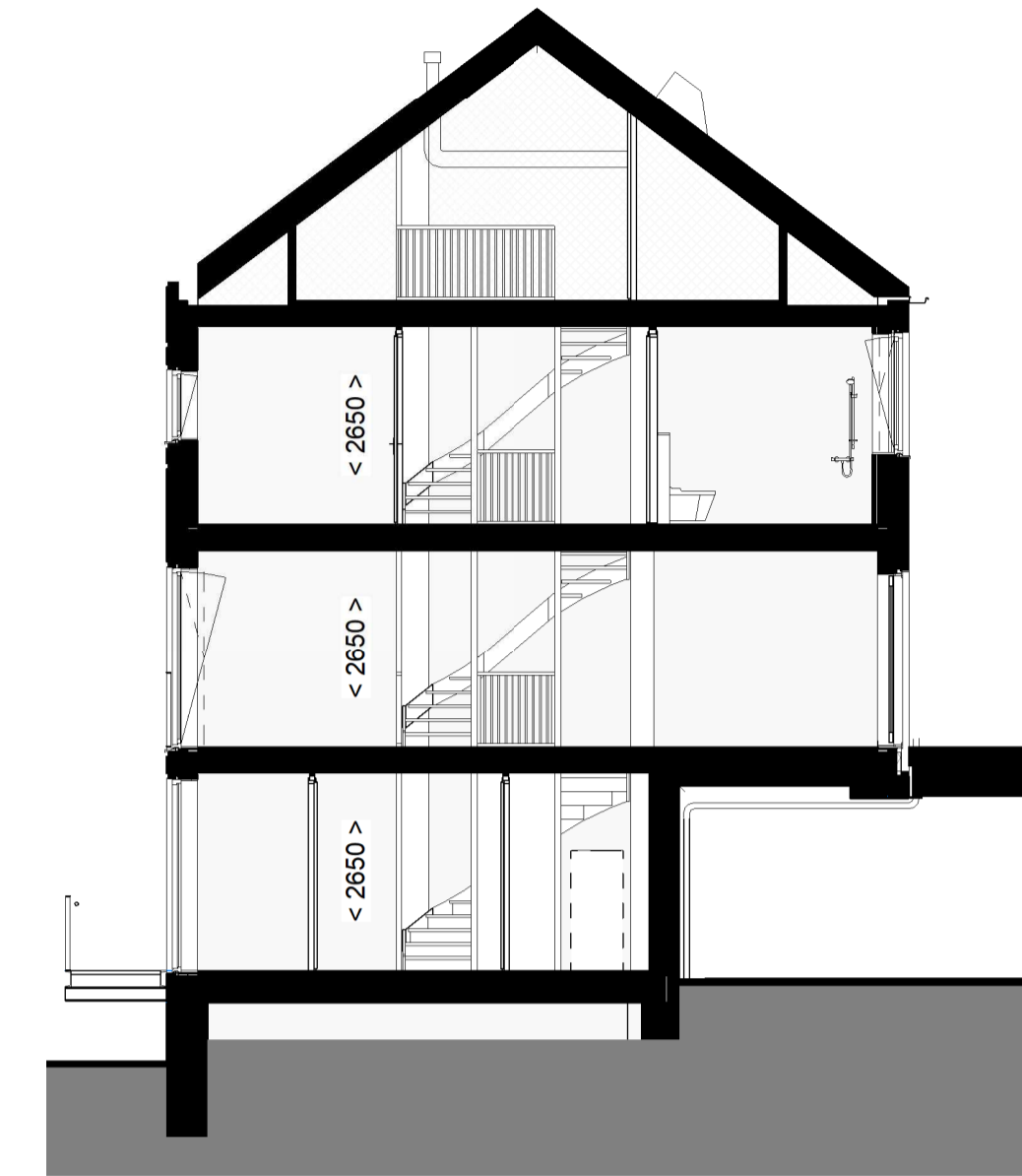
1:100 DOORSNEDE
