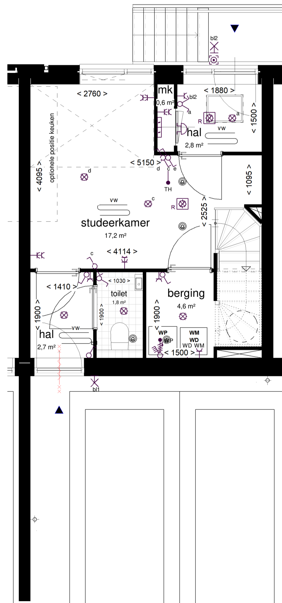
1:50 BEGANE GROND
