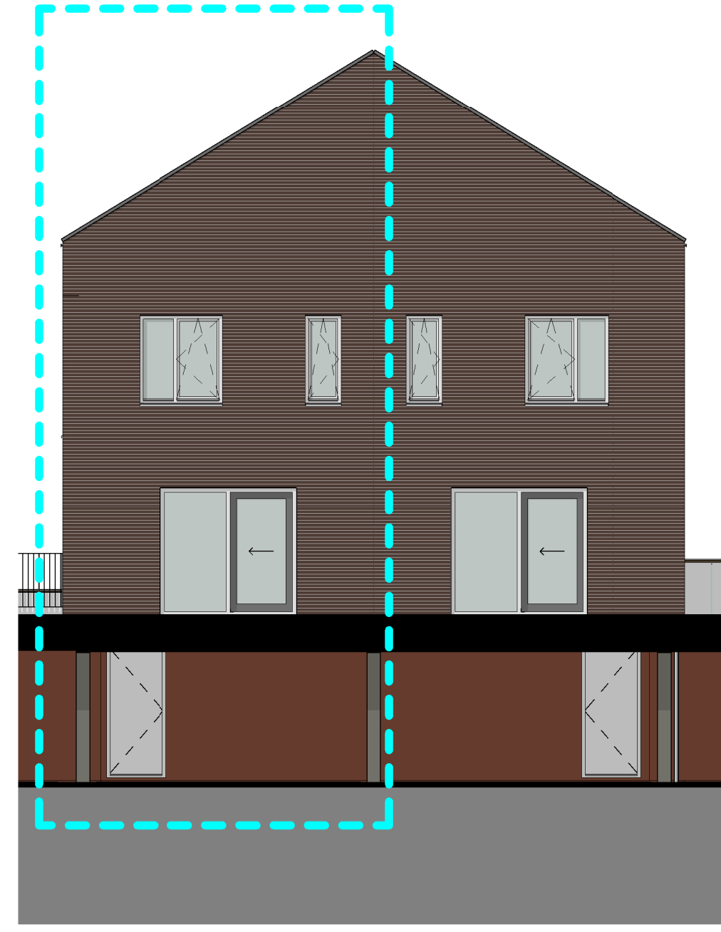
1:100 ACHTERGEVEL (ZUID)
