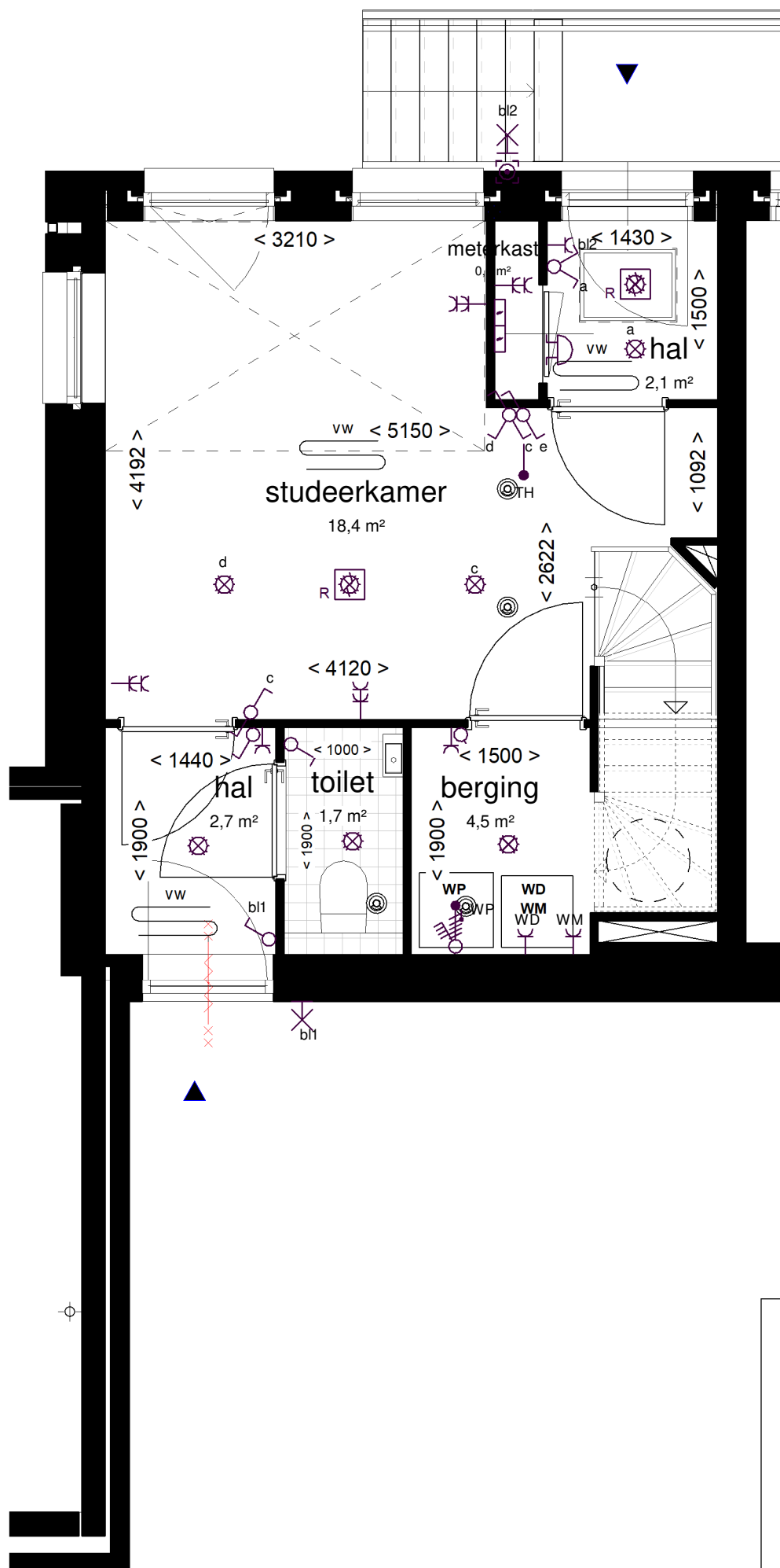
1:50 BEGANE GROND
