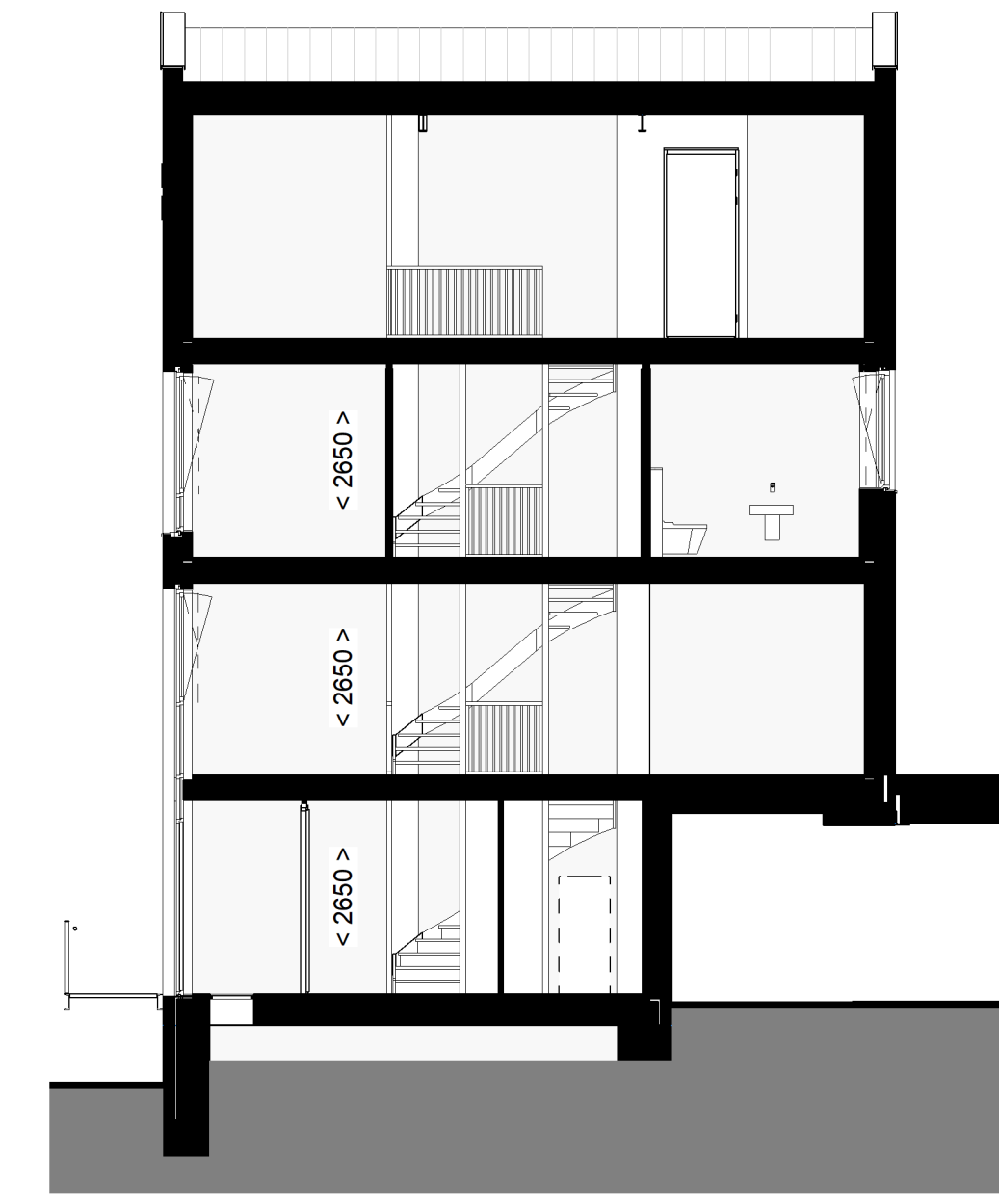
1:100 DOORSNEDE
