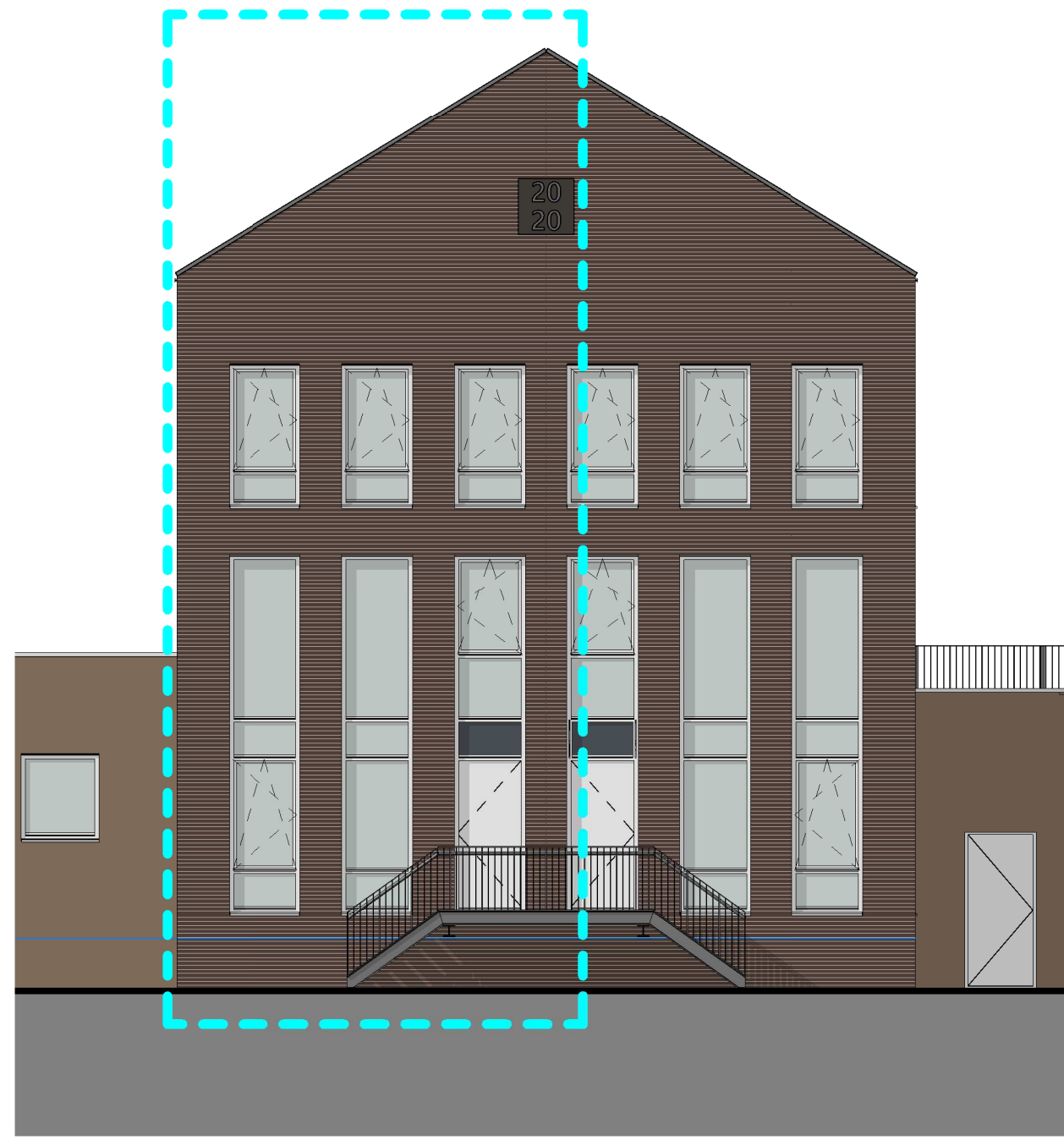
1:100 VOORGEVEL (NOORD)
