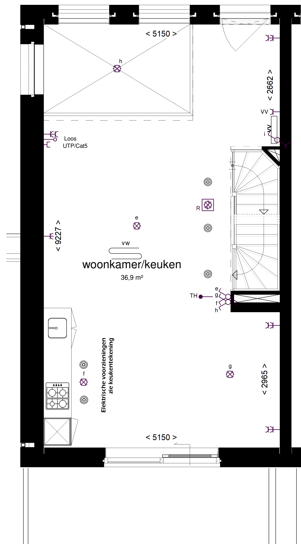
1:50 1e VERDIEPING
