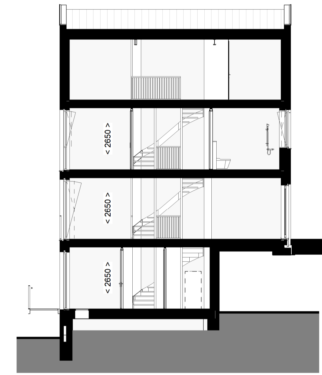
1:100 DOORSNEDE
