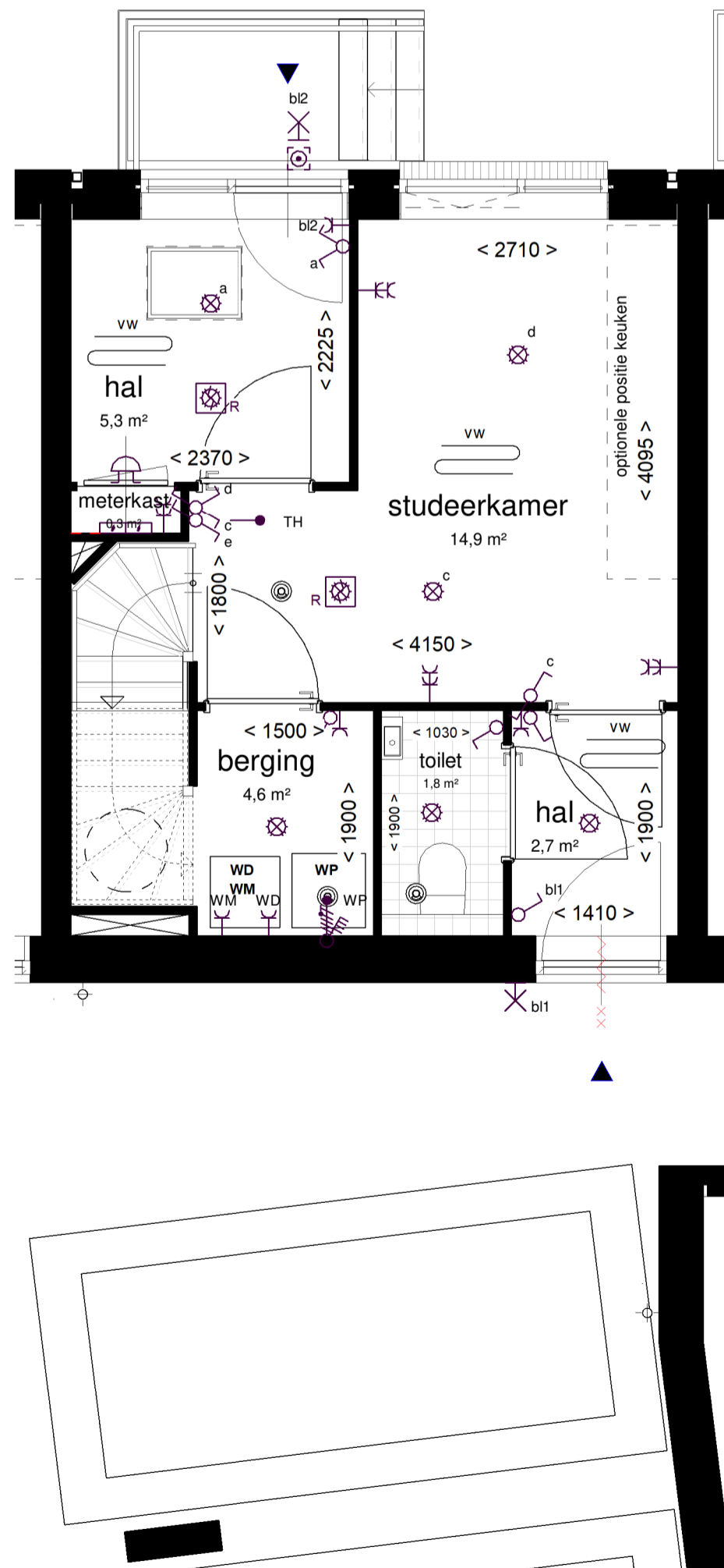
1:50 BEGANE GROND
