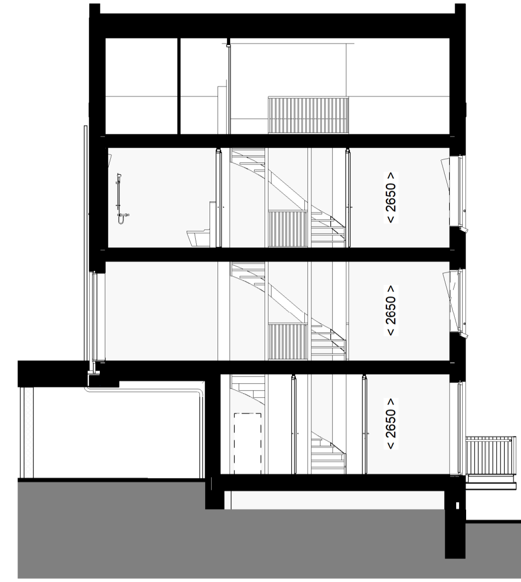
1:100 DOORSNEDE
