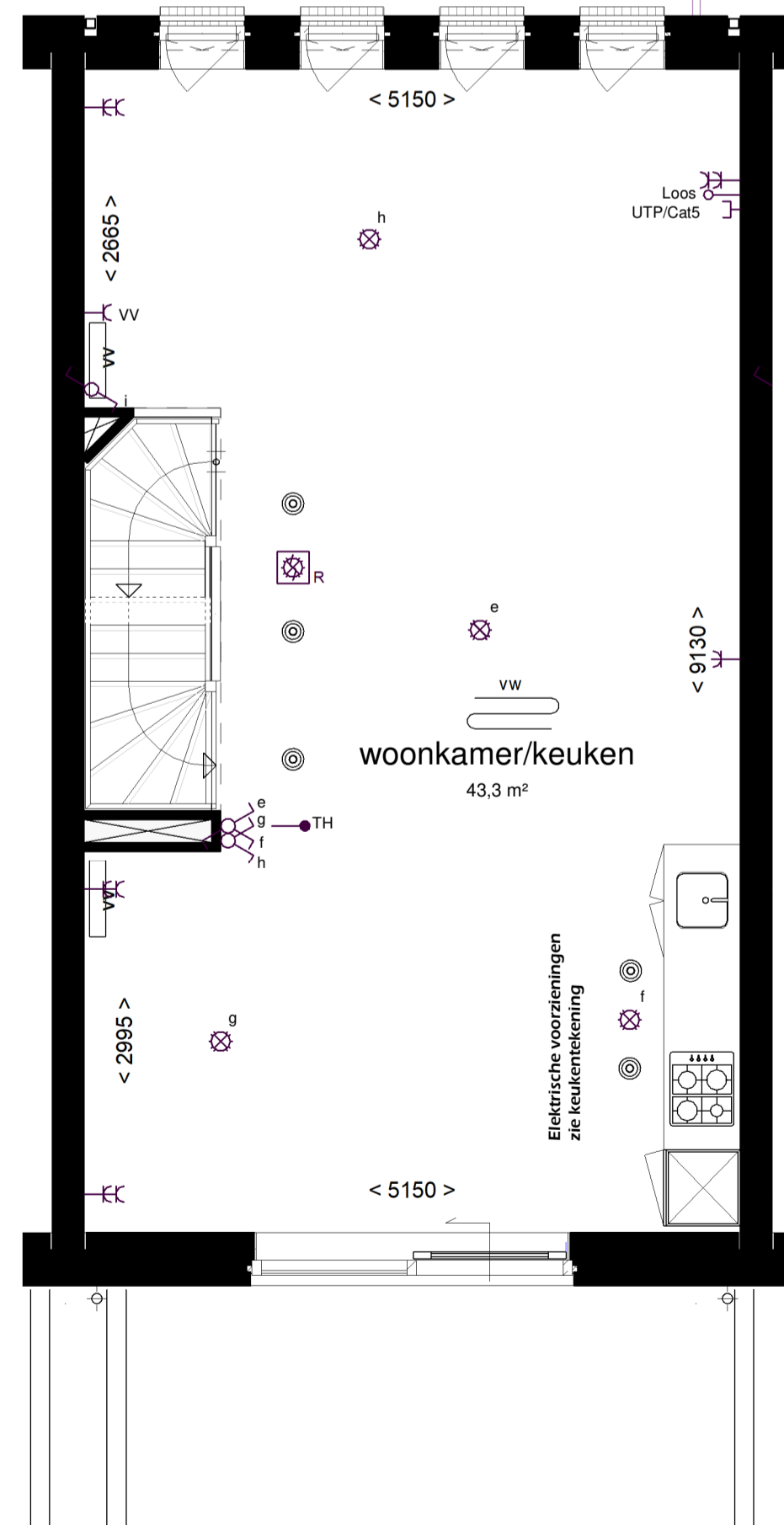
1:50 1e VERDIEPING
