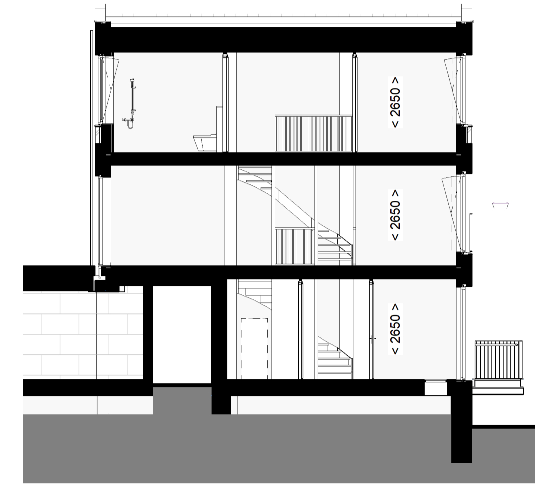
DOORSNEDE 1:100
