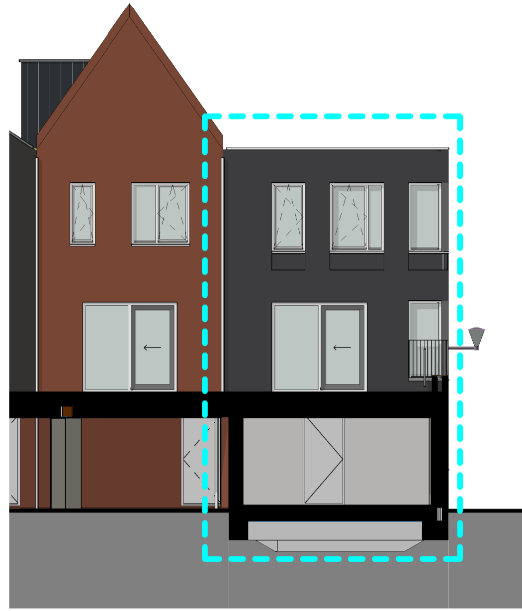
ACHTERGEVEL (WEST)
