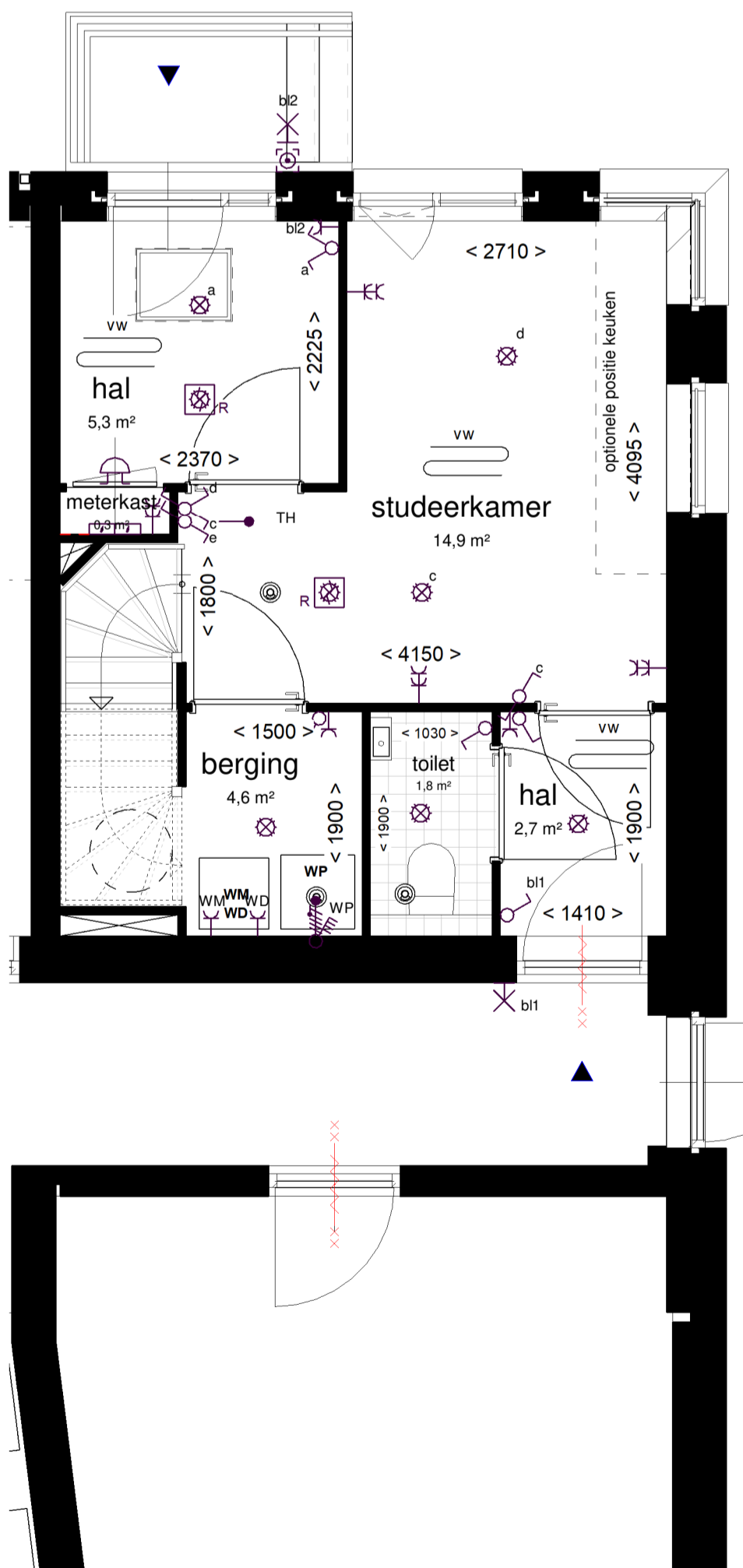
1:50 BEGANE GROND
