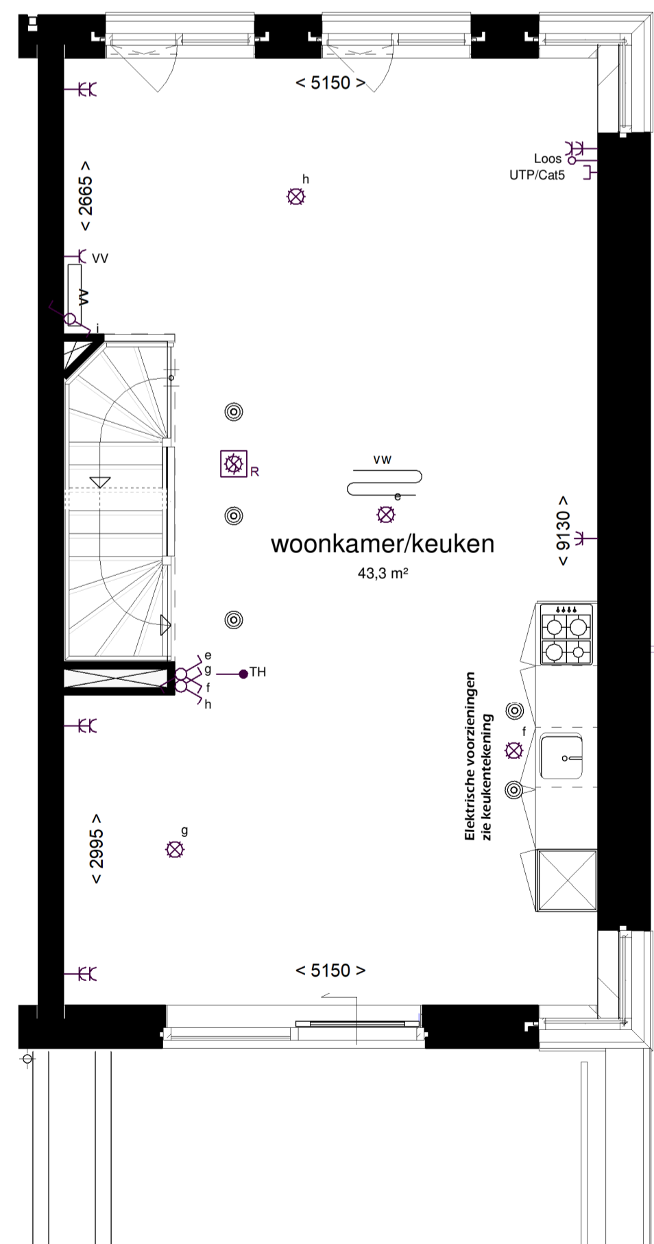
1:50 1e VERDIEPING
