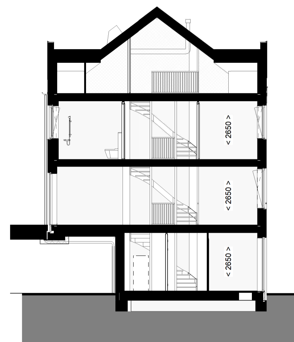
1:100 DOORSNEDE
