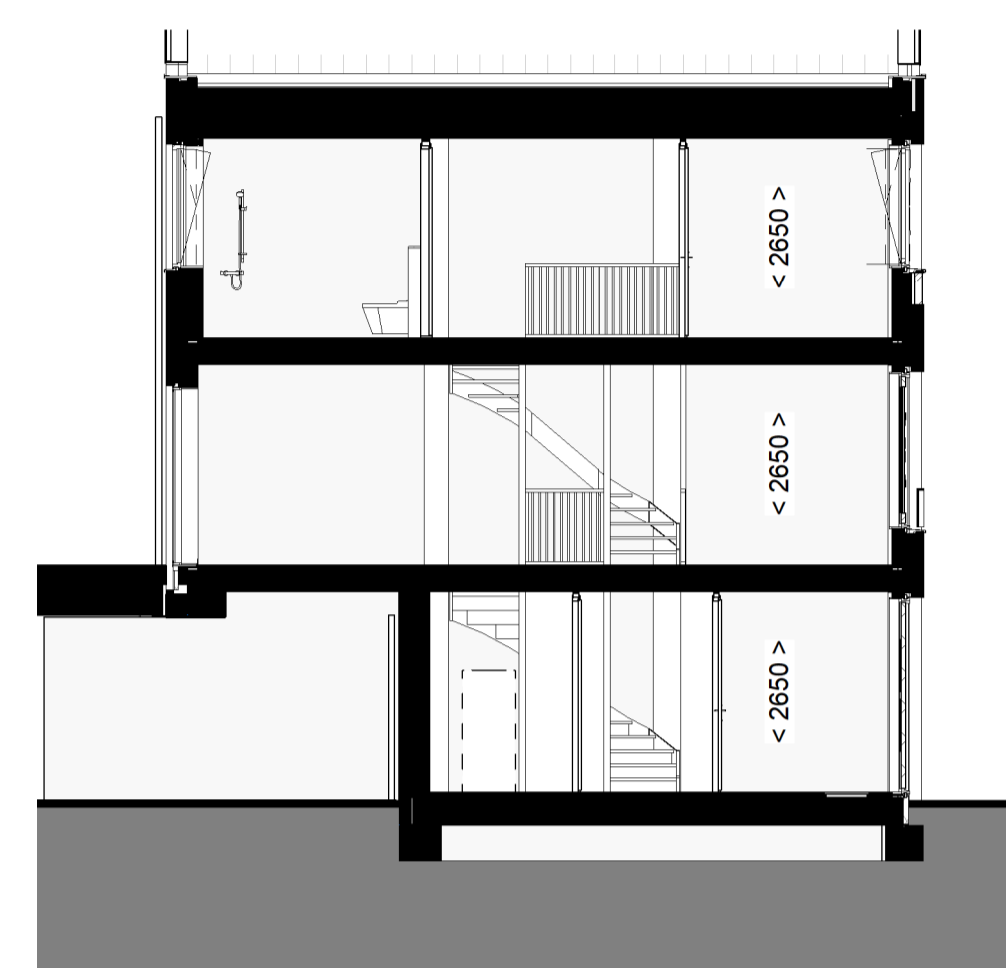
1 : 100 DOORSNEDE
