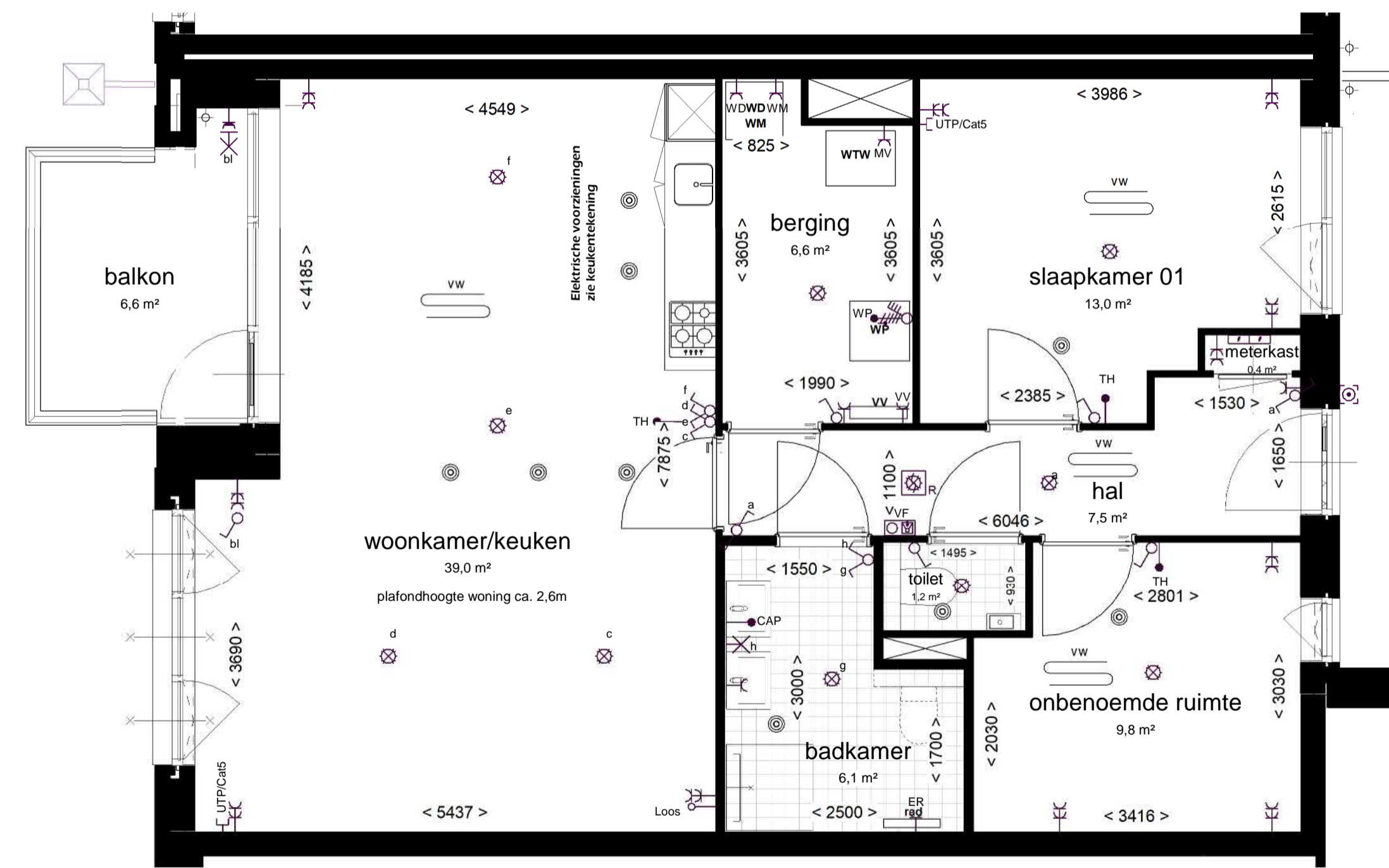
1: 50 PLATTEGROND
