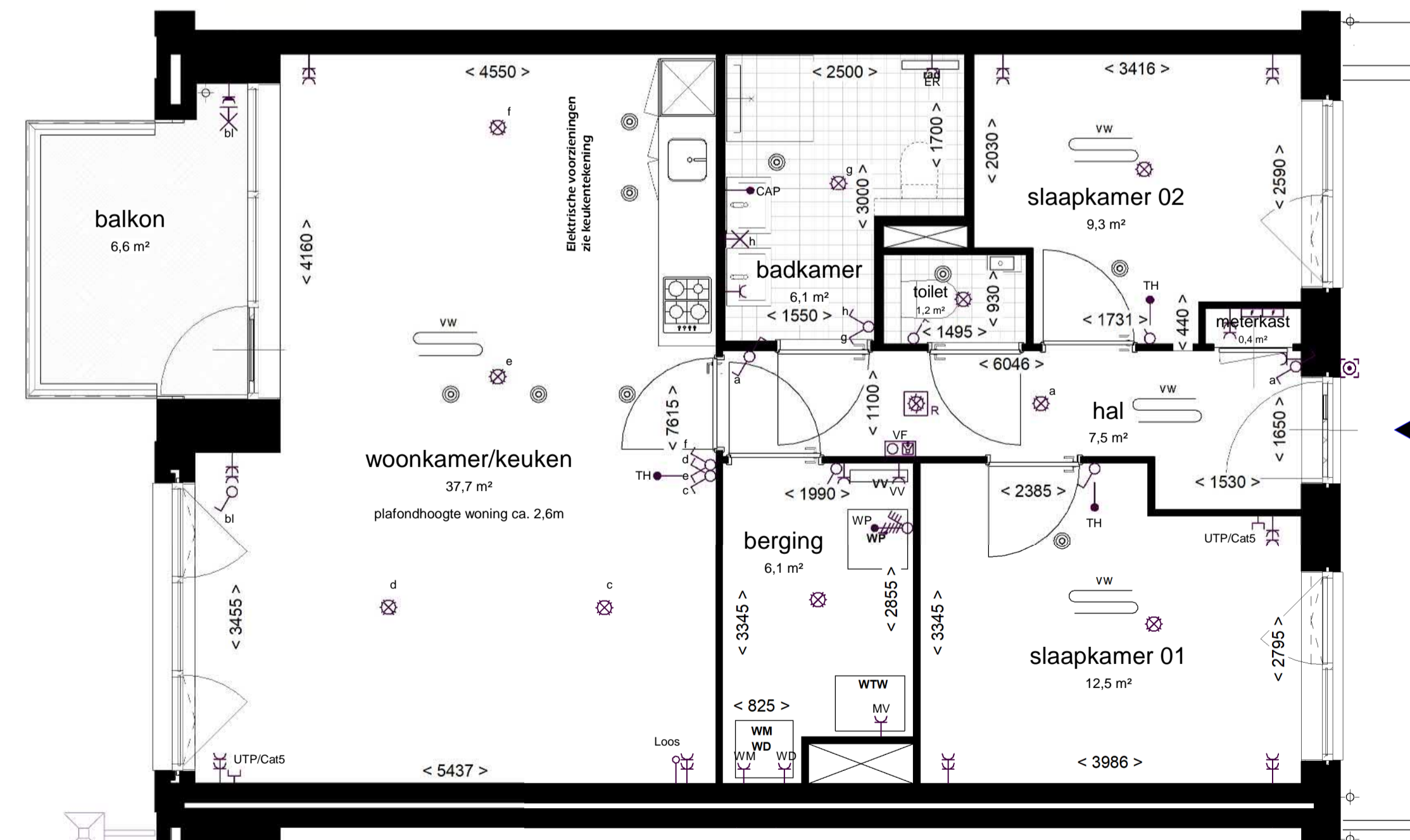
1:50 PLATTEGROND
