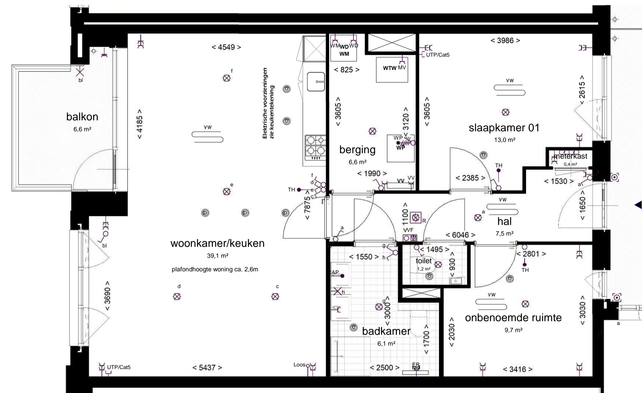
1:50 PLATTEGROND
