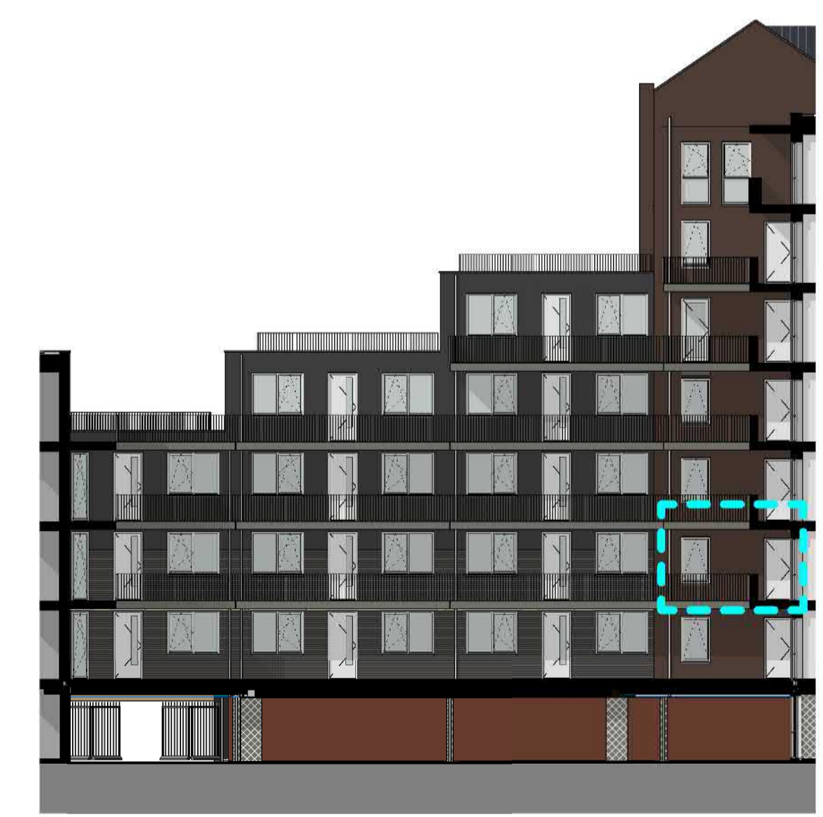
1:200 ZIJGEVEL (OOST)
