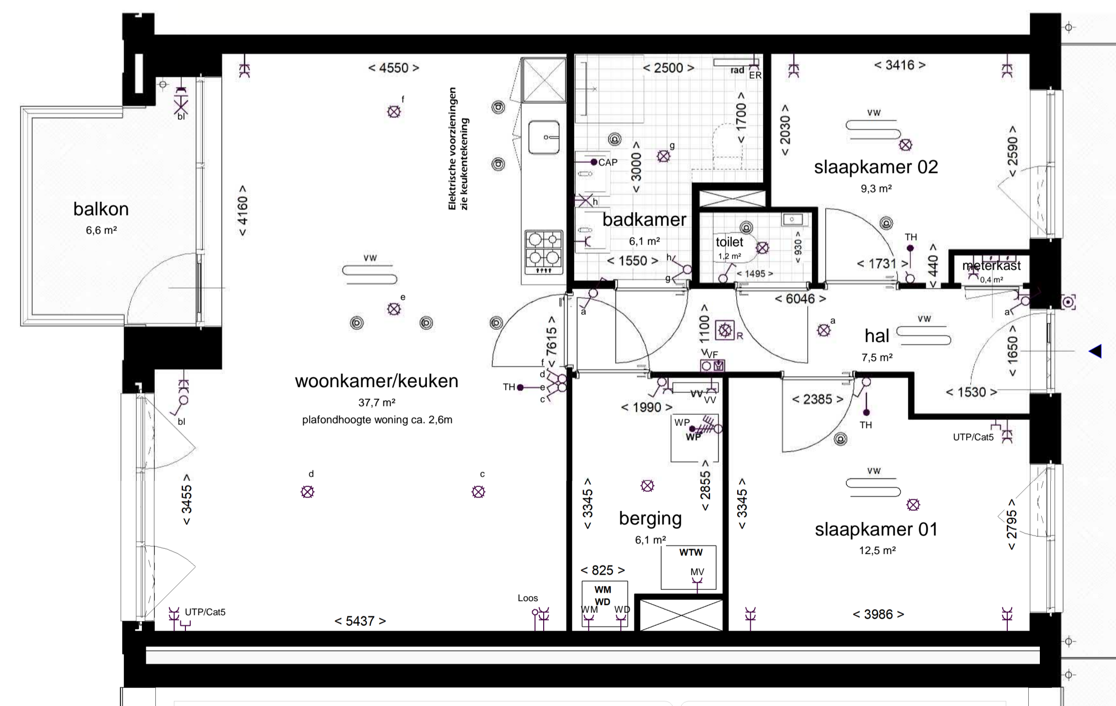
1:50 PLATTEGROND
