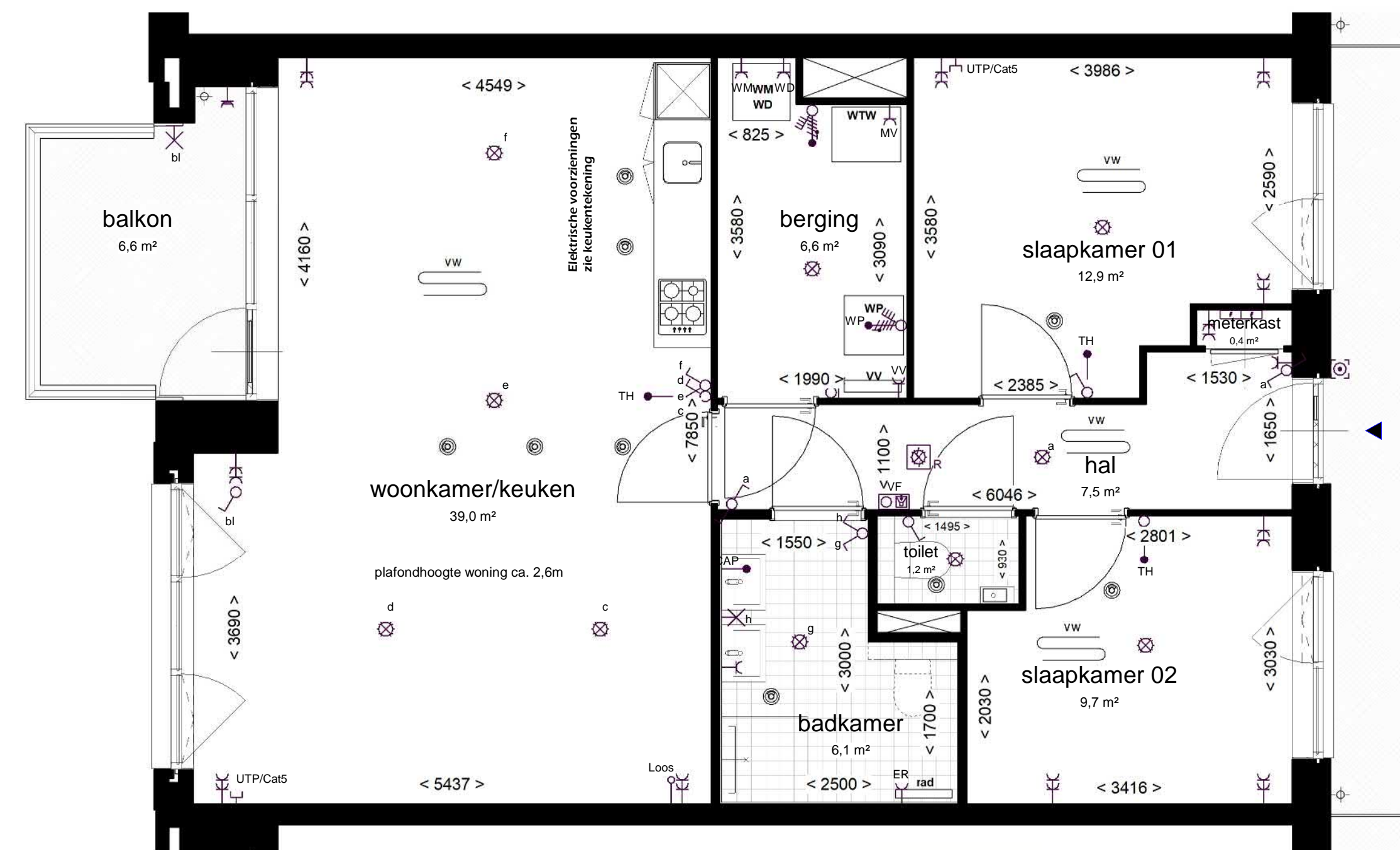
1: 50 PLATTEGROND
