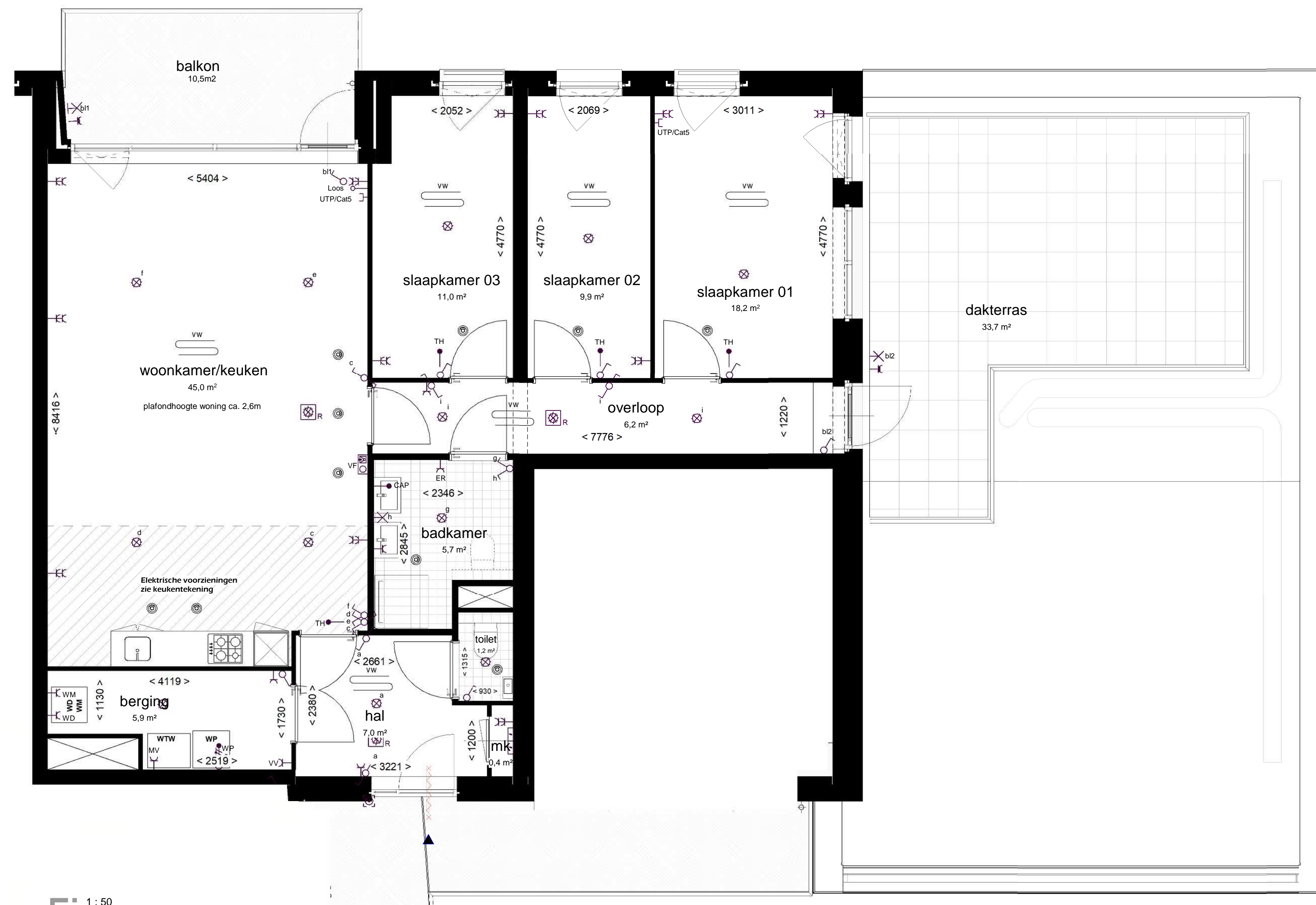
1:50 PLATTEGROND
