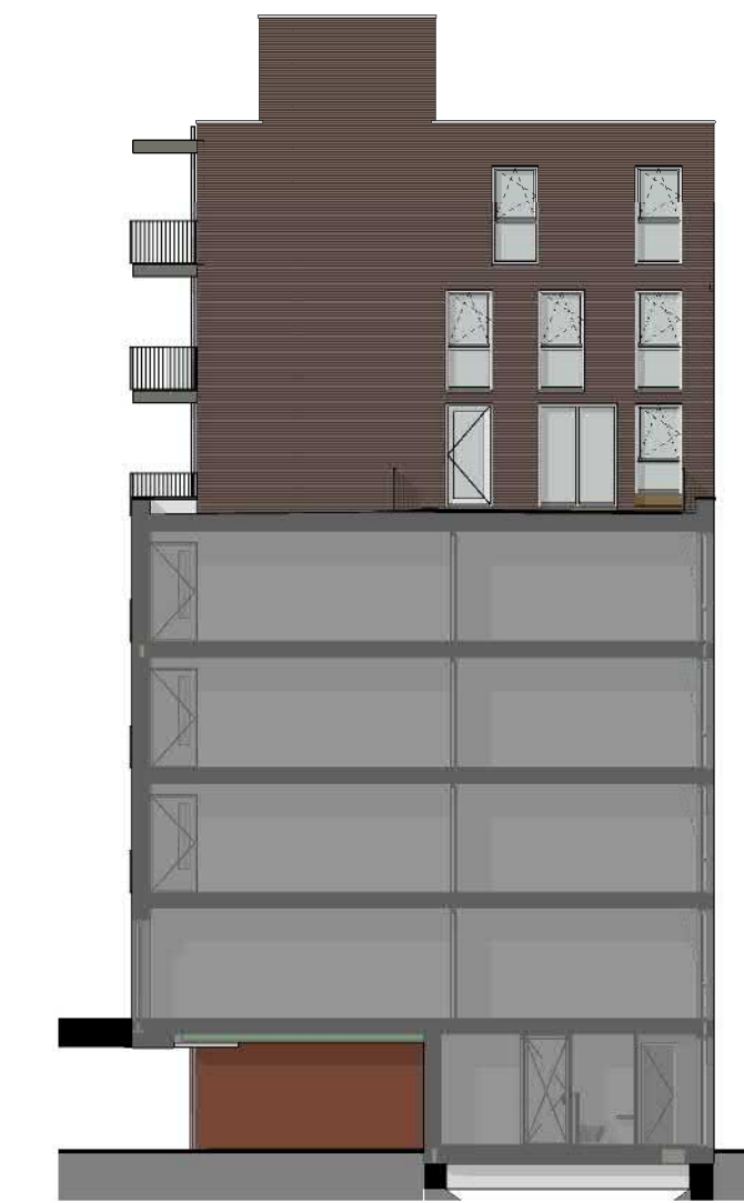
1:200 ZIJGEVEL (OOST)
