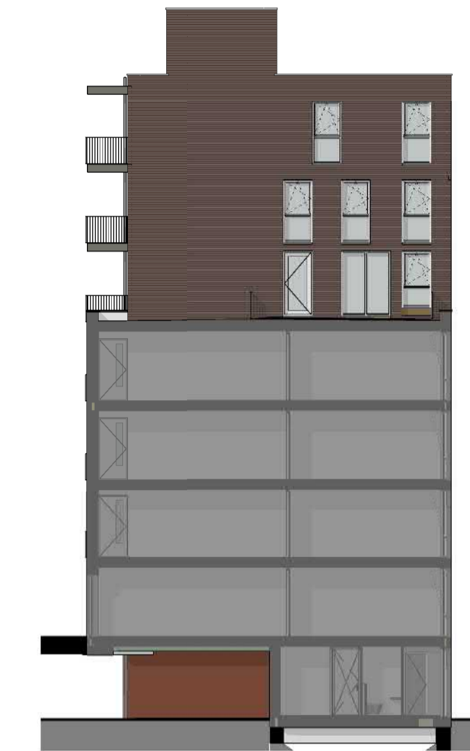
1:200 ZIJGEVEL (OOST)
